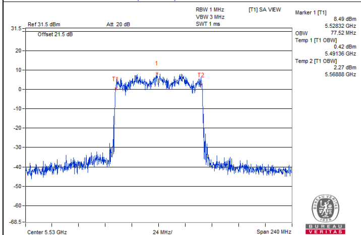
802.11ax (HE80+80) / Chain 1 : CH 106+122(L)
