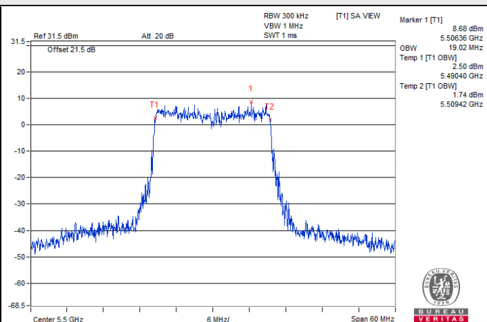
802.11ax (HE20) / Chain 1 : CH 100
