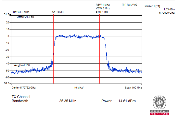
802.11n (HT40) CDD / Chain 0 : CH 142 (U-NII-2C)
