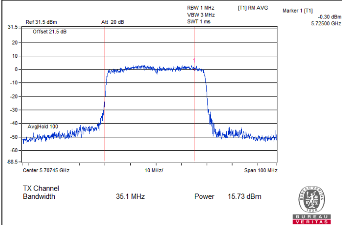
802.11n (HT40) CDD / Chain 1 : CH 142 (U-NII-2C)
