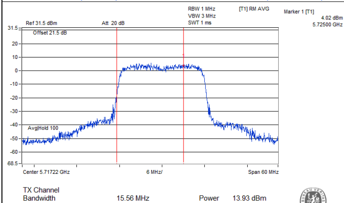
802.11n (HT40) CDD / Chain 3 : CH 142 (U-NII-2C)
