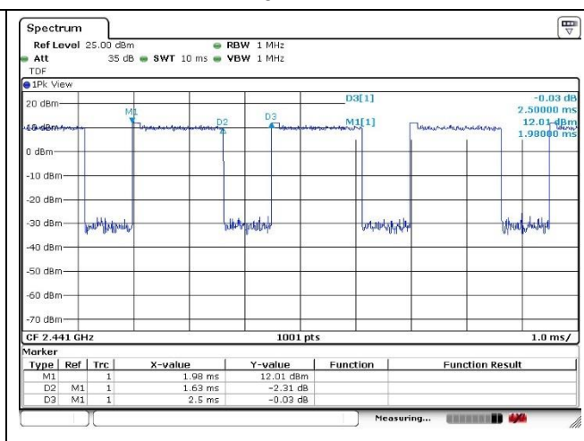
8DPSK
