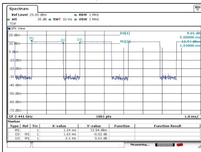
GFSK
