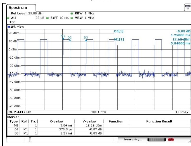
GFSK
