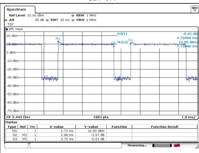
8DPSK
