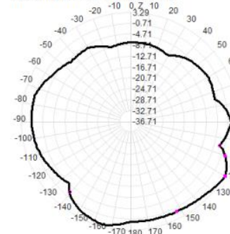
2465.0MHz Total(E2-YZ), Max= 3.29dBi
