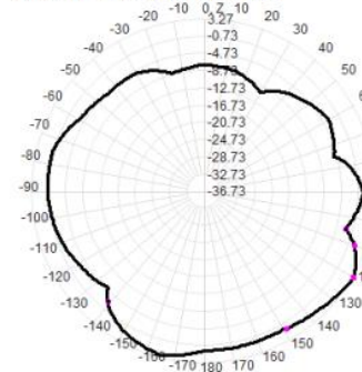
2475.0MHz Total(E2-YZ), Max= 3.27dBi
