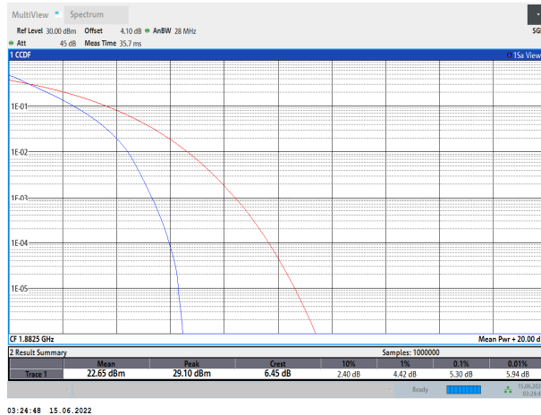
Band25-20MHz-QPSK-26365-100RB#0
