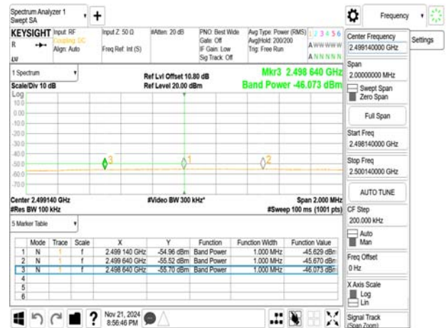
802.11ax_20MHz_2457MHz_RU52_40
