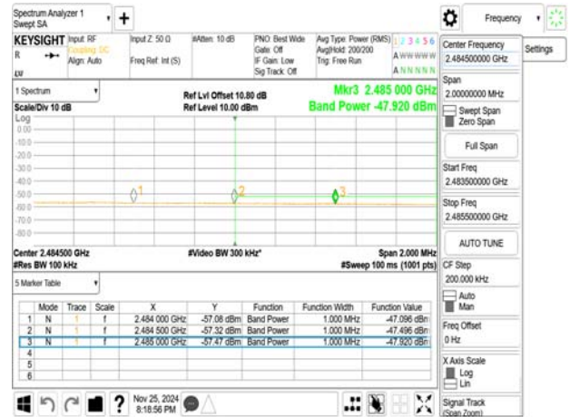
802.11ax_20MHz_2457MHz_RU26_8
