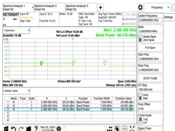
802.11ax_20MHz_2412MHz
