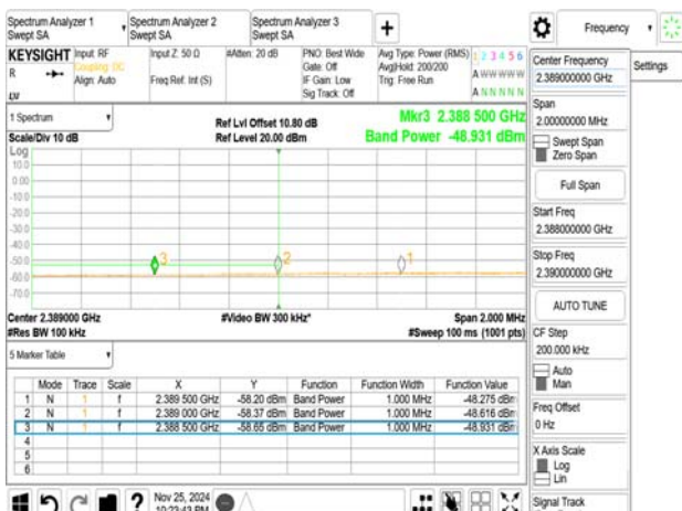
802.11ax_20MHz_2437MHz_RU242_L
