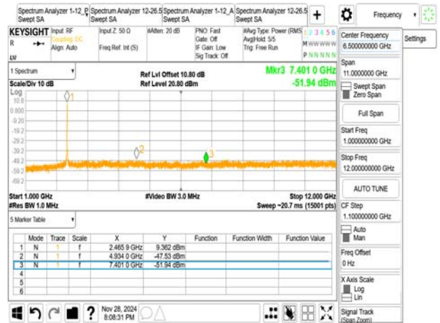
802.11b_20MHz_2472MHz
