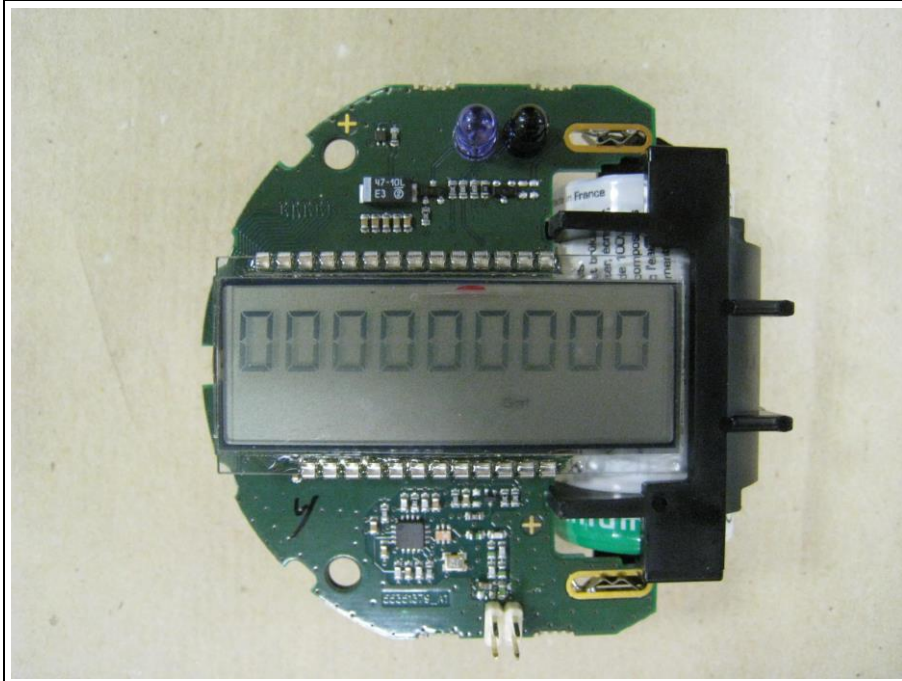
PCB TOP
