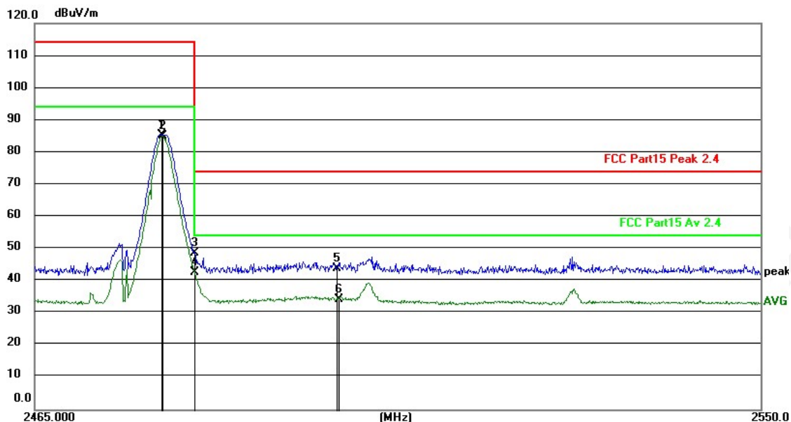
2480MHz Horizontal
