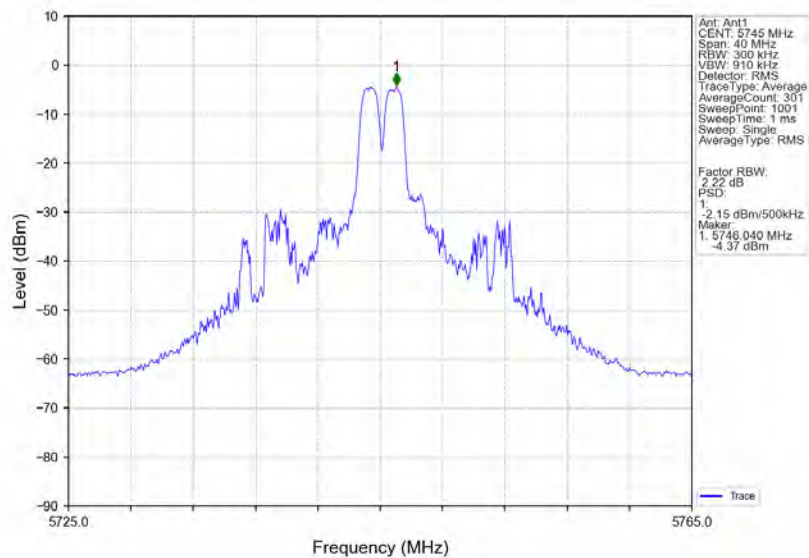
802.11ax(HE20) LCH 5745MHz RU26 Mid Ant1 NTN
