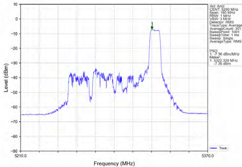
802.11ax(HE80) MCH 5290MHz RU106 Right MIMO NTVN
