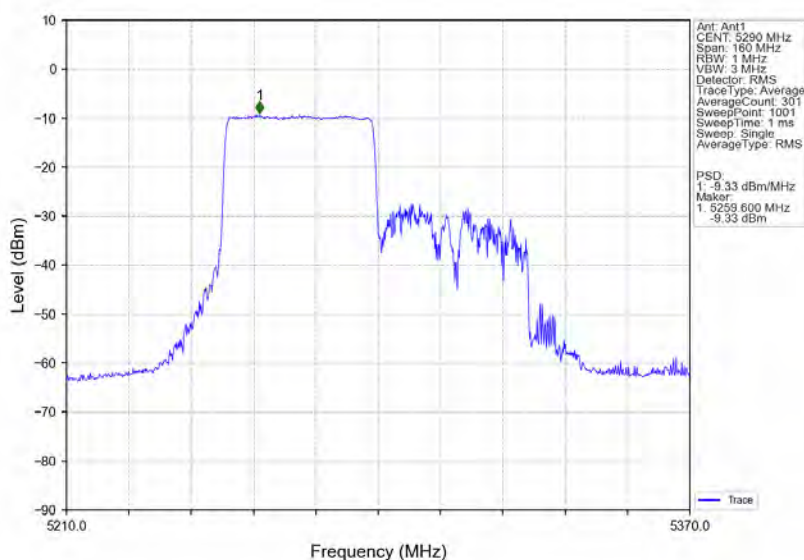
802.11ax(HE80) MCH 5290MHz RU484 Left Ant1 NTN
