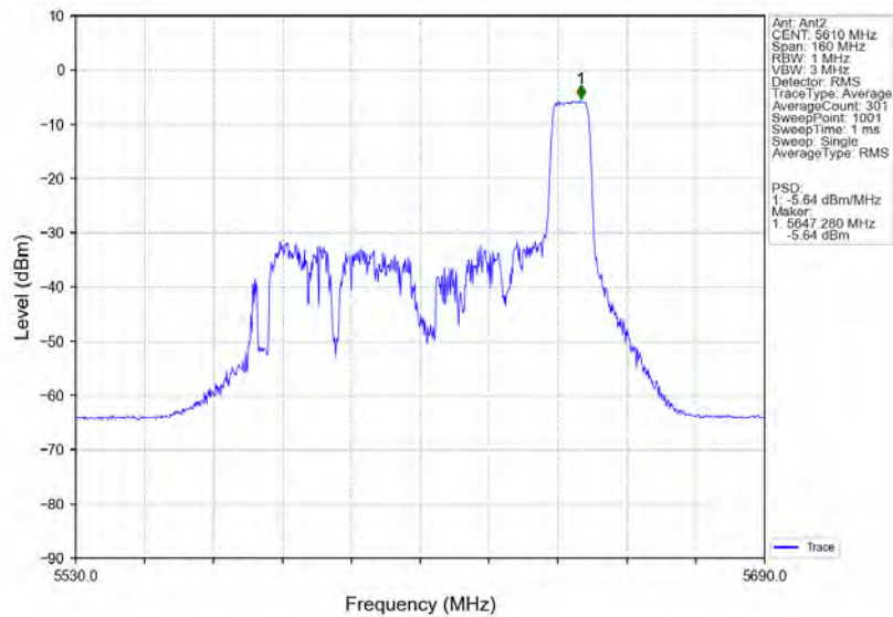
802.11ax(HE80) HCH 5610MHz RU106 Right MIMO NTN
