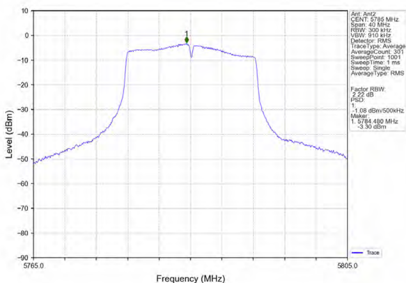
802.11a MCH 5785MHz MIMO NTN
