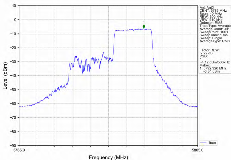
802.11ax(HE20) MCH 5785MHz RU106 Right Ant2 NTVN
