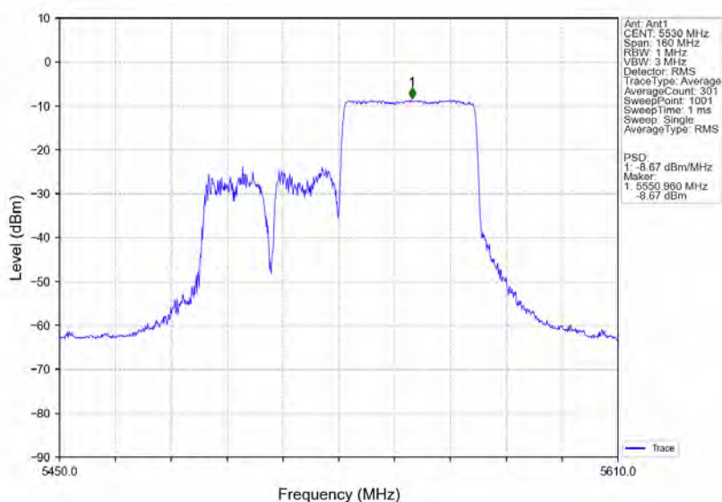
802.11ax(HE80) LCH 5530MHz RU484 Right Ant1 NTVN
