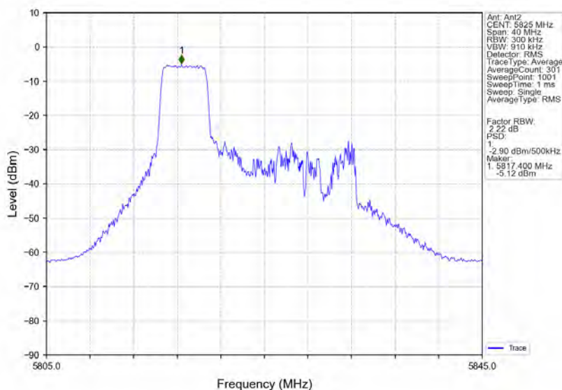
802.11ax(HE20) HCH 5825MHz RU52 Left MIMO NTN
