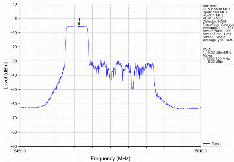
802.11ax(HE80) LCH 5530MHz RU242 Left MIMO NTN
