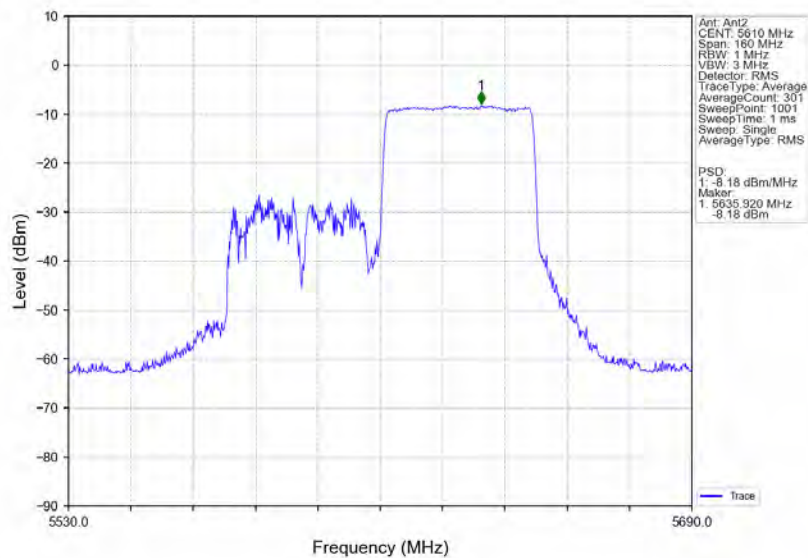
802.11ax(HE80) HCH 5610MHz RU484 Right Ant2 NTV
