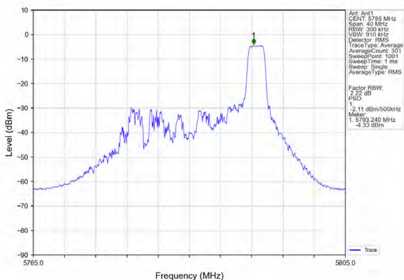
802.11ax(HE20) MCH 5785MHz RU26 Right Ant1 NTN
