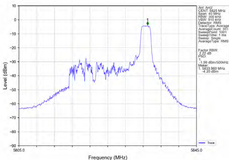
802.11ax(HE20) HCH 5825MHz RU26 Right Ant2 NTNv
