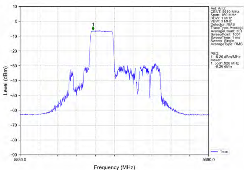
802.11ax(HE80) HCH 5610MHz RU242 Mid MIMO NTNv
