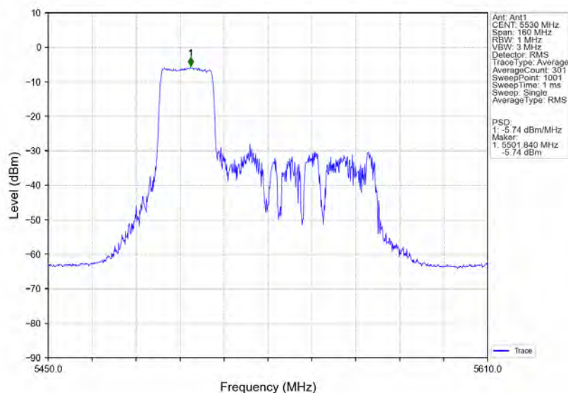
802.11ax(HE80) LCH 5530MHz RU242 Left Ant1 NTN
