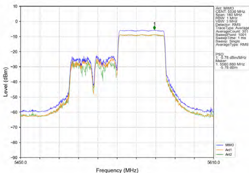
802.11ax(HE80) LCH 5530MHz RU484 Right MIMO NTVN
