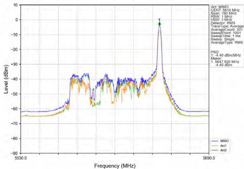
802.11ax(HE80) HCH 5610MHz RU26 Right MIMO NTNv
