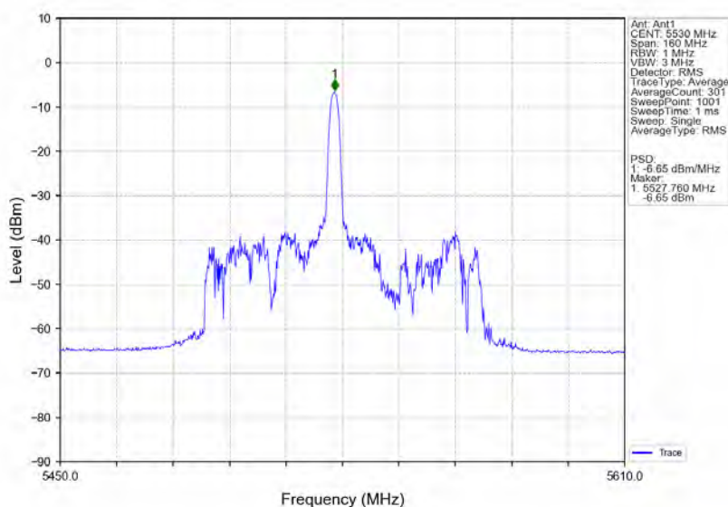
802.11ax(HE80) LCH 5530MHz RU26 Mid Ant1 NTN
