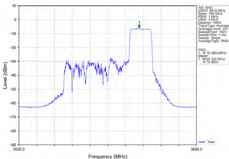
802.11ax(HE80) HCH 5610MHz RU242 Right Ant2 NTV
