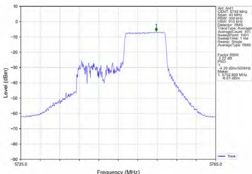
802.11ax(HE20) LCH 5745MHz RU106 Right Ant1 NTV
