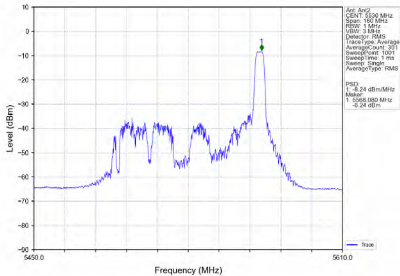
802.11ax(HE80) LCH 5530MHz RU52 Right MIMO NTN
