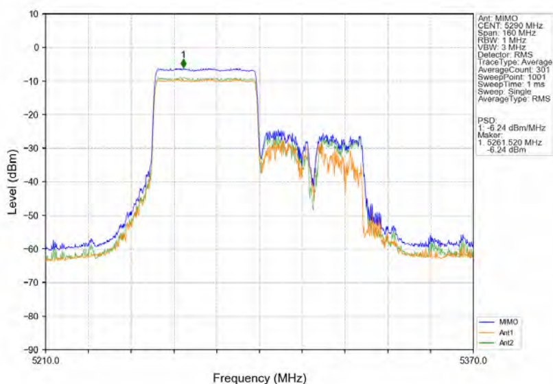
802.11ax(HE80) MCH 5290MHz RU484 Left MIMO NTNv
