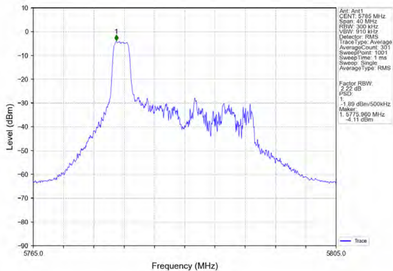
802.11ax(HE20) MCH 5785MHz RU26 Left Ant1 NTN
