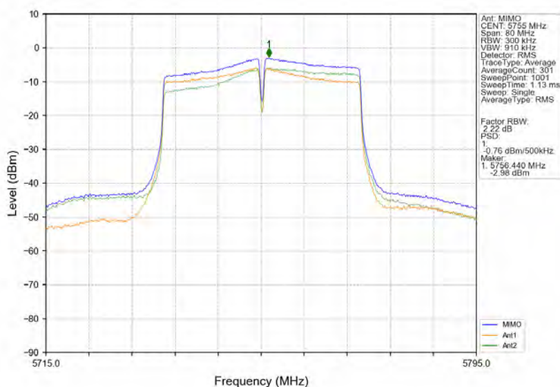
802.11ac(VHT40) LCH 5755MHz MIMO NTN
