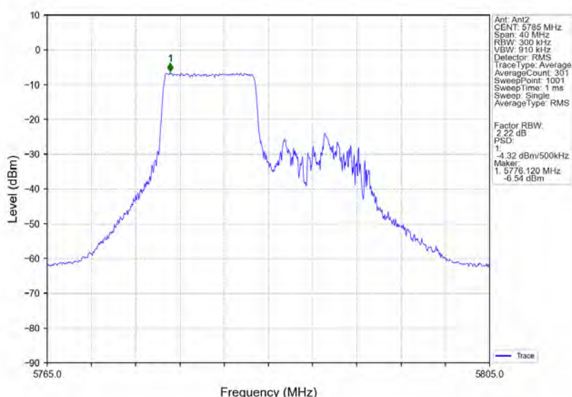
802.11ax(HE20) MCH 5785MHz RU106 Left MIMO NTN
