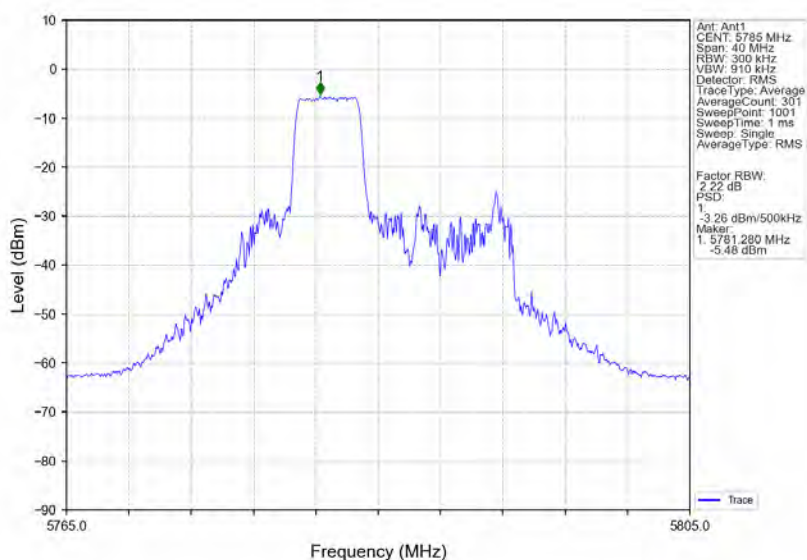
802.11ax(HE20) MCH 5785MHz RU52 Mid Ant1 NTNv
