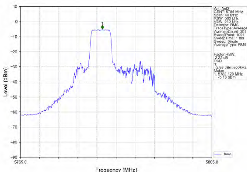
802.11ax(HE20) MCH 5785MHz RU52 Mid MIMO NTN
