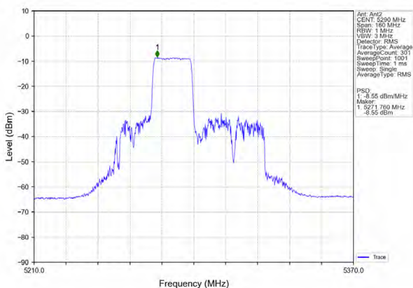
802.11ax(HE80) MCH 5290MHz RU242 Mid MIMO NTN
