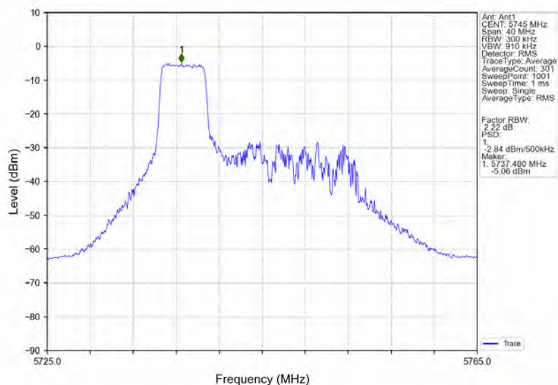
802.11ax(HE20) LCH 5745MHz RU52 Left Ant1 NTN
