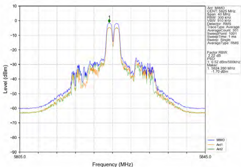
802.11ax(HE20) HCH 5825MHz RU26 Mid MIMO NTN
