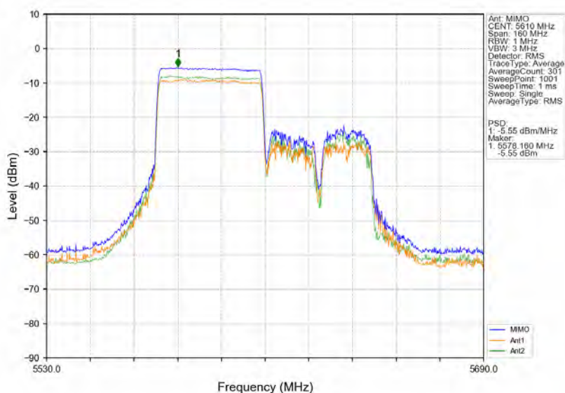
802.11ax(HE80) HCH 5610MHz RU484 Left MIMO NTN
