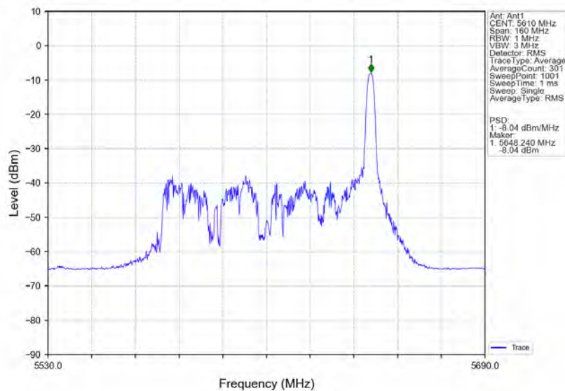
802.11ax(HE80) HCH 5610MHz RU26 Right Ant1 NTN
