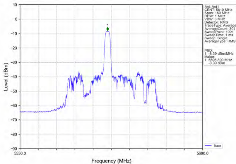
802.11ax(HE80) HCH 5610MHz RU52 Mid Ant1 NTNv
