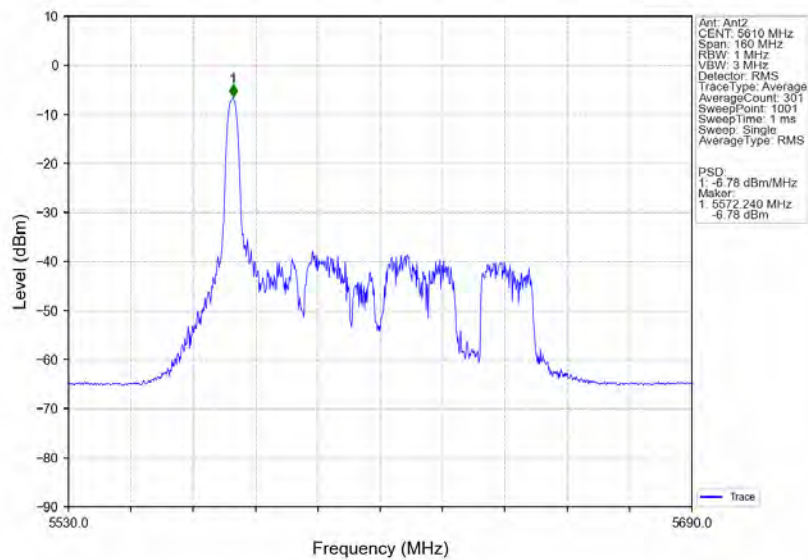
802.11ax(HE80) HCH 5610MHz RU26 Left MIMO NTN
