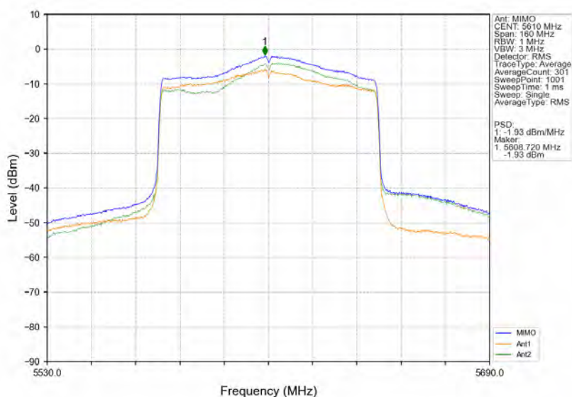
802.11ax(HE80) HCH 5610MHz RU996 Left MIMO NTN
