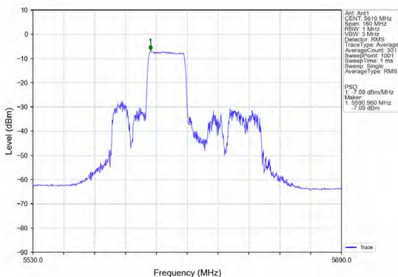
802.11ax(HE80) HCH 5610MHz RU242 Mid Ant1 NTN
