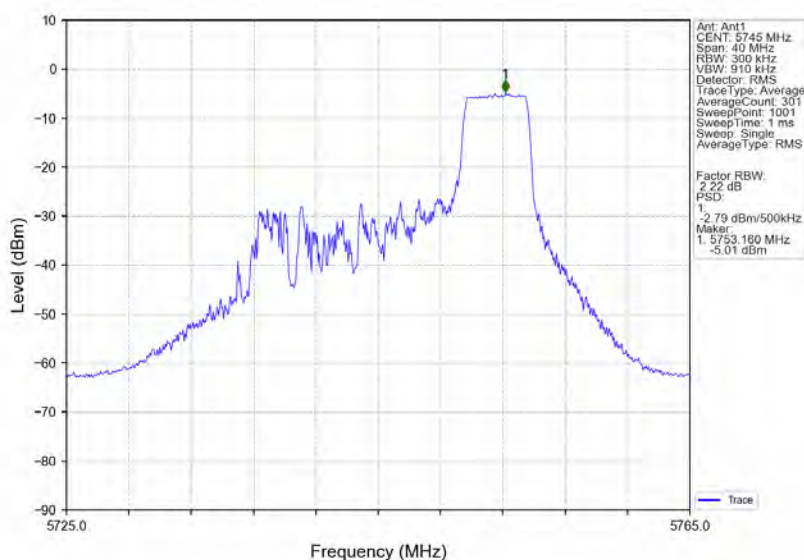
802.11ax(HE20) LCH 5745MHz RU52 Right Ant1 NTNv
