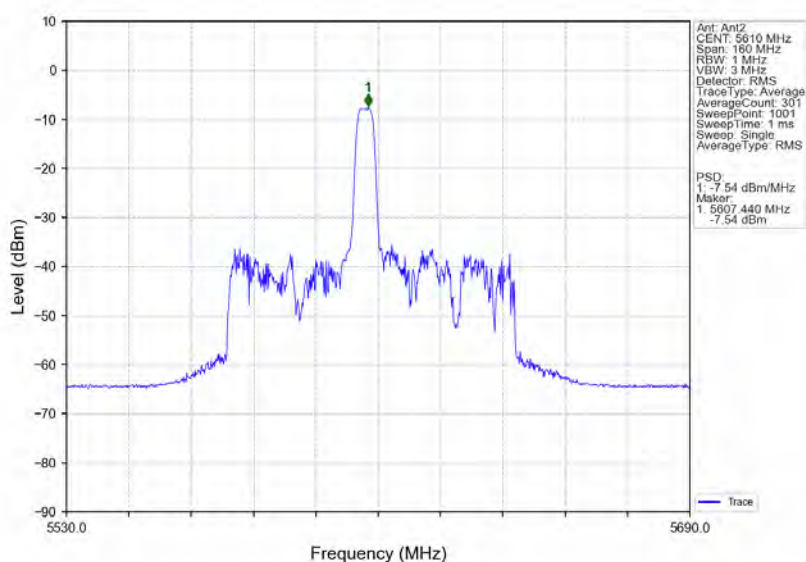
802.11ax(HE80) HCH 5610MHz RU52 Mid MIMO NTN
