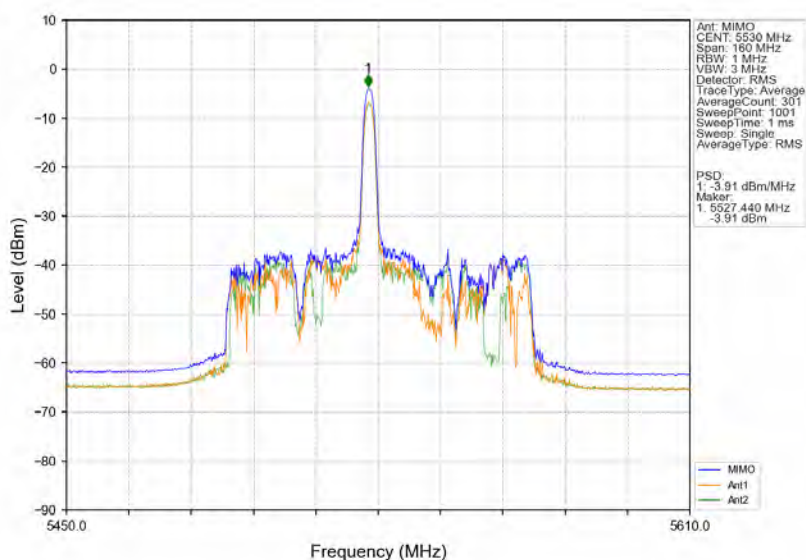
802.11ax(HE80) LCH 5530MHz RU26 Mid MIMO NTN
