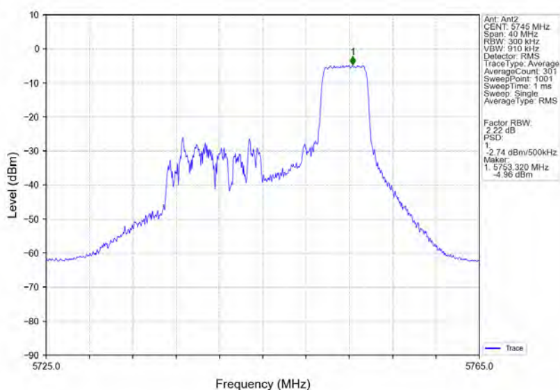
802.11ax(HE20) LCH 5745MHz RU52 Right MIMO NTNv
