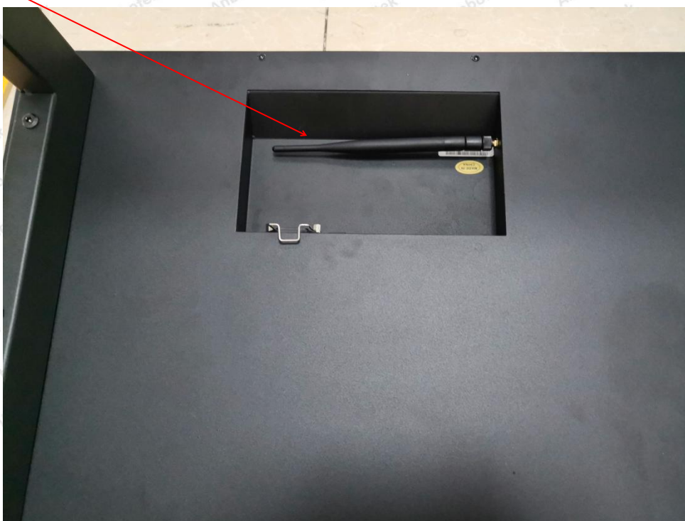
BLE&WIFI ANT
