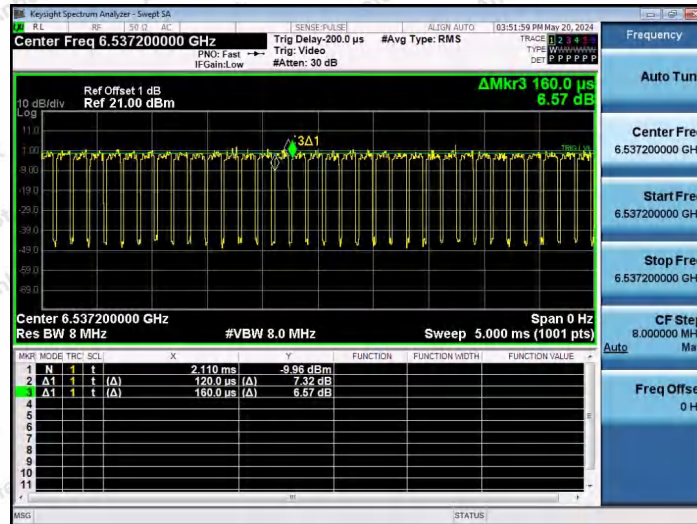
NTNV-11AX80SISO-Ant1-6545-484Tone-RU65
