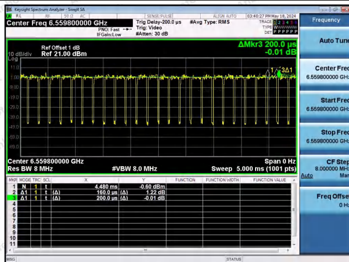
NTNV-11AX40SISO-Ant1-6565-242Tone-RU61
