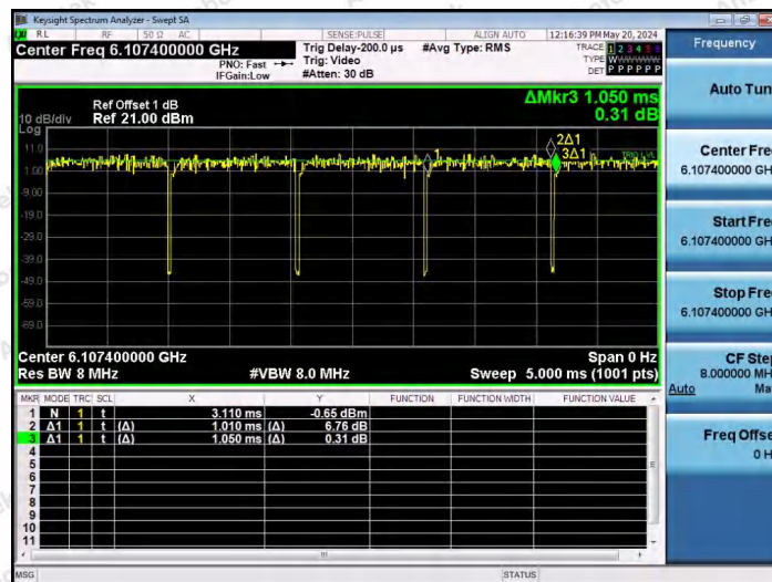
NTNV-11AX80SISO-Ant1-6145-26Tone-RU0
