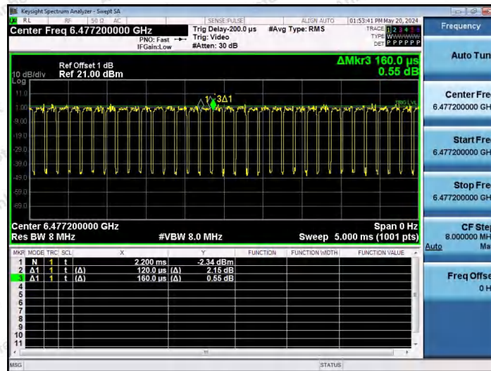
NTNV-11AX80SISO-Ant1-6465-484Tone-RU66
