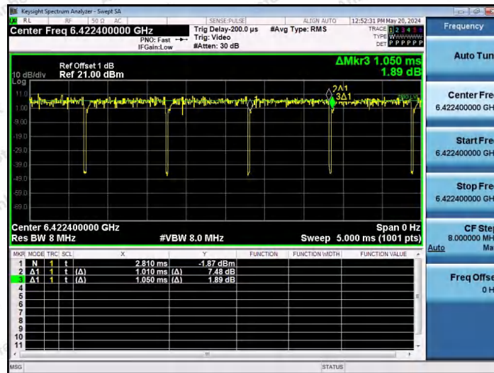
NTNV-11AX80SISO-Ant1-6385-26Tone-RU36
