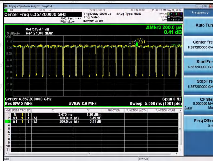
NTNV-11AX80SISO-Ant1-6385-242Tone-RU61
