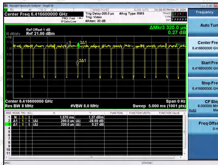
NTNV-11AX80SISO-Ant1-6385-106Tone-RU60
