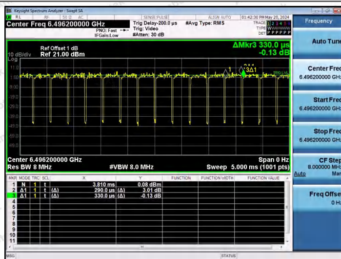
NTNV-11AX80SISO-Ant1-6465-106Tone-RU60
