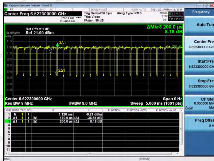
NTNV-11AX40SISO-Ant1-6525-242Tone-RU61
