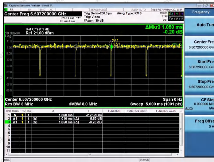
NTNV-11AX80SISO-Ant1-6507-200Tone-RU66
