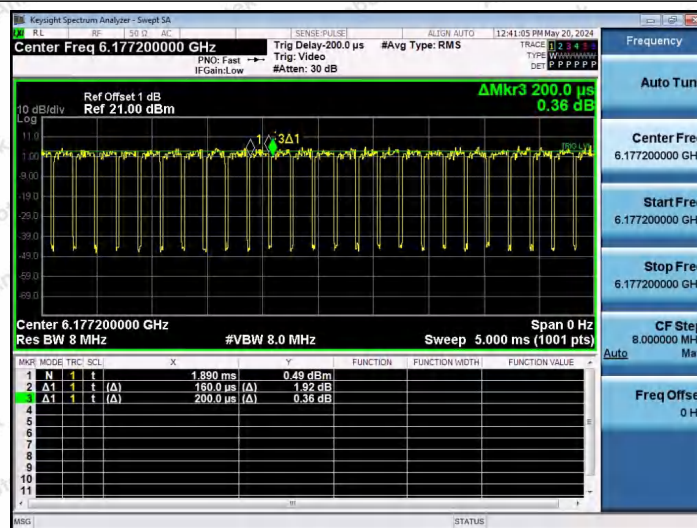
NTNV-11AX80SISO-Ant1-6145-242Tone-RU64
