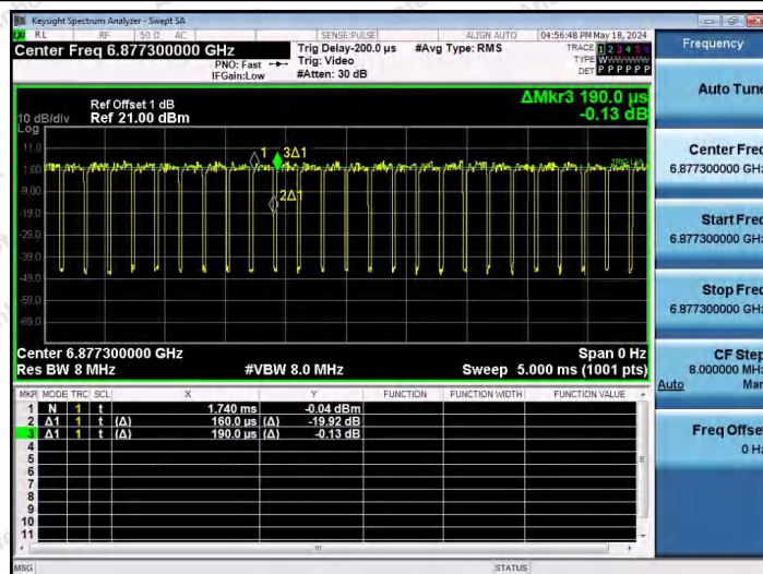
NTNV-11AX40SISO-Ant1-6885-242Tone-RU61
