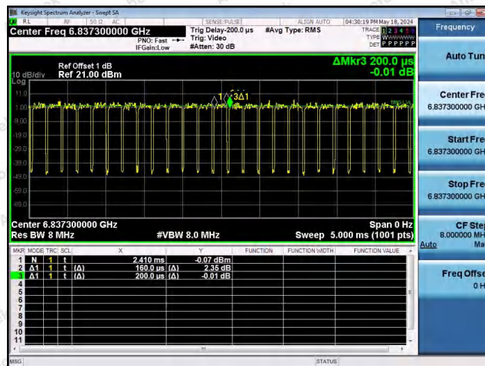
NTNV-11AX40SISO-Ant1-6845-242Tone-RU61
