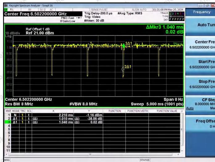
NTNV-11AX80SISO-Ant1-6465-26Tone-RU36
