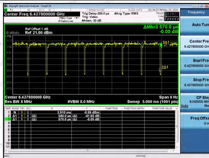
NTNV-11AX80SISO-Ant1-6465-52Tone-RU37
