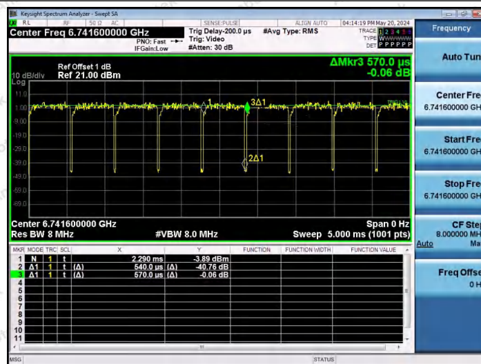
NTNV-11AX80SISO-Ant1-6705-52Tone-RU52
