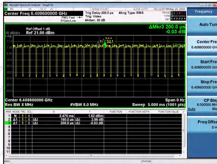
NTNV-11AX80SISO-Ant1-6385-242Tone-RU64
