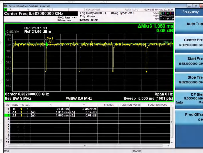
NTNV-11AX80SISO-Ant1-6582-000Tone-RU66
