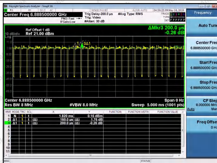
NTNV-11AX40SISO-Ant1-6885-242Tone-RU62
