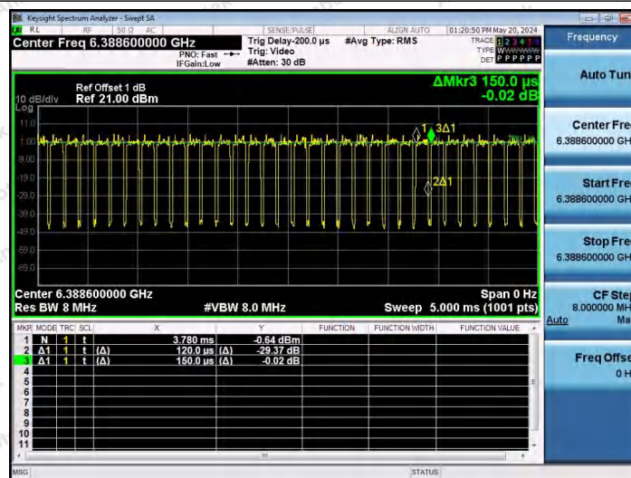
NTNV-11AX80SISO-Ant1-6385-484Tone-RU66
