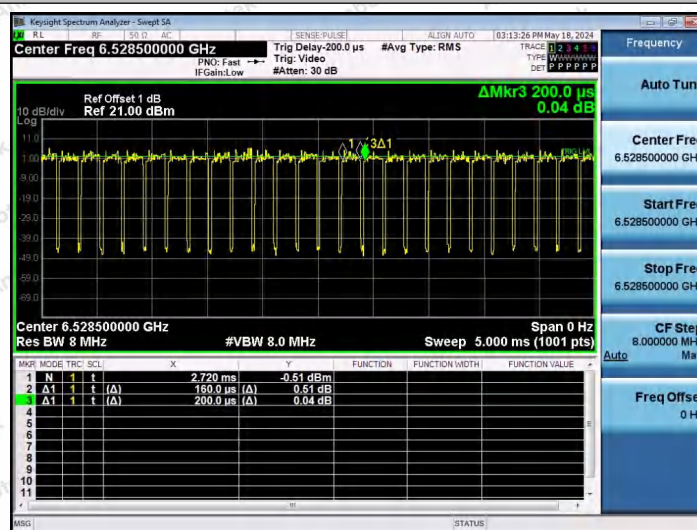
NTNV-11AX40SISO-Ant1-6525-242Tone-RU62
