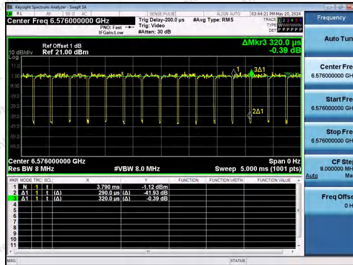
NTNV-11AX80SISO-Ant1-6545-106Tone-RU60
