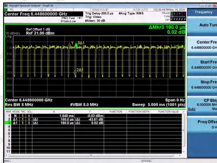
NTNV-11AX40SISO-Ant1-6445-242Tone-RU62
