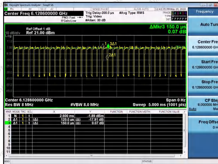
NTNV-11AX80SISO-Ant1-6145-484Tone-RU65
