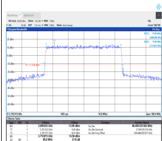
1-N77-3700-3980--30-90-L-3-DFT-16QAM-O
