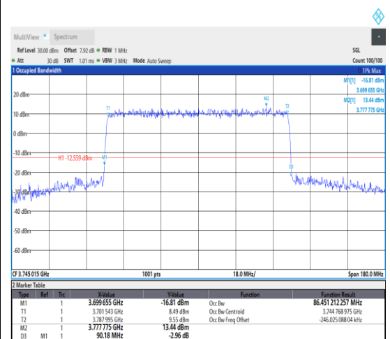
1-N77-3700-3980--30-90-L-4-DFT-64QAM-O
