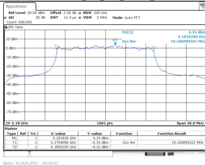
11AX20MIMO_Ant2_5180_242Tone_RU61
