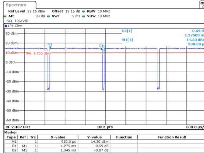
11B_Ant1_2437
