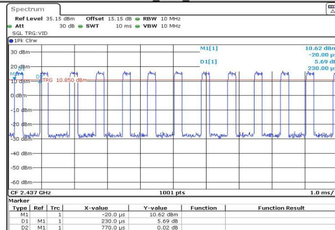
11G_Ant1_2437
