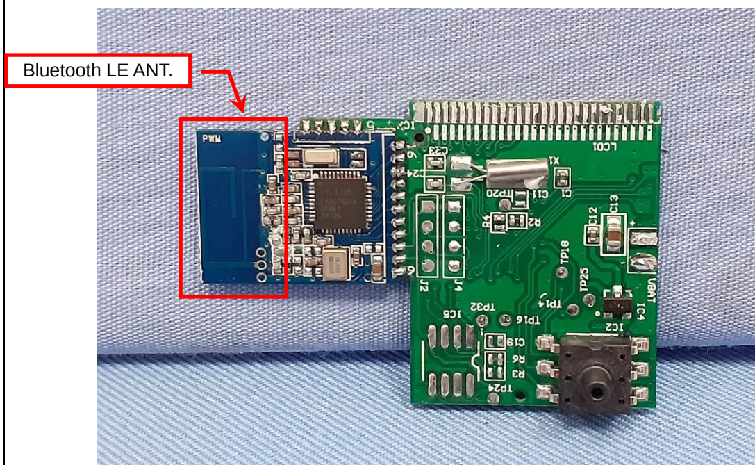
EUT Photo (10)
