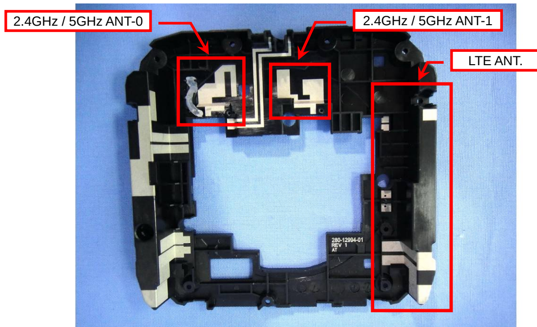
EUT Photo (16)
