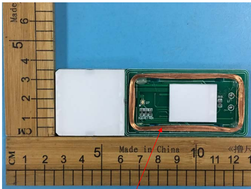
Antenna
