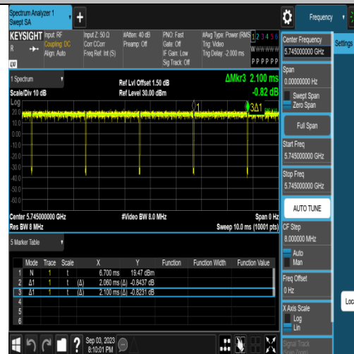
NTNV-11A-Ant1-5745
