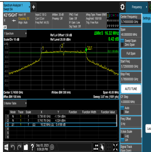
11A-Ant1-5745
