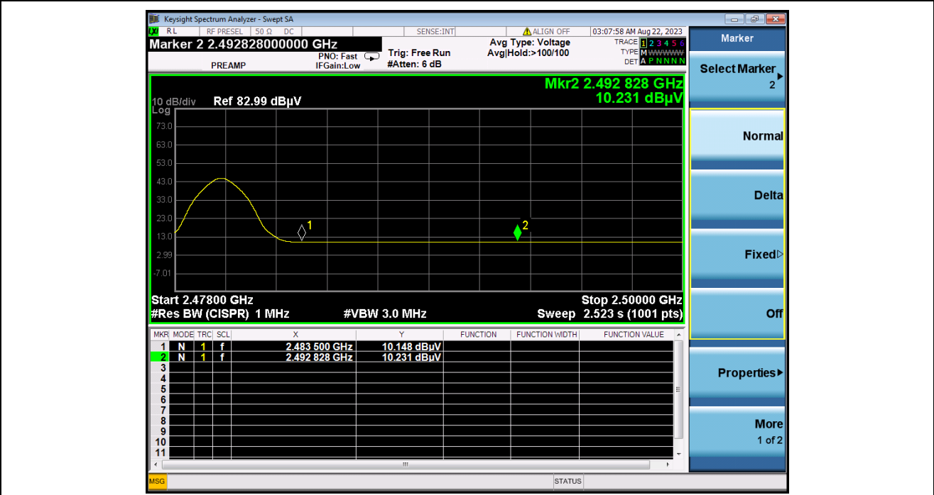
(AVERAGE, Channel 39)
