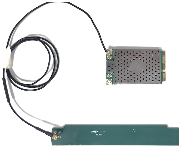
RFID Coupler and RFID module
