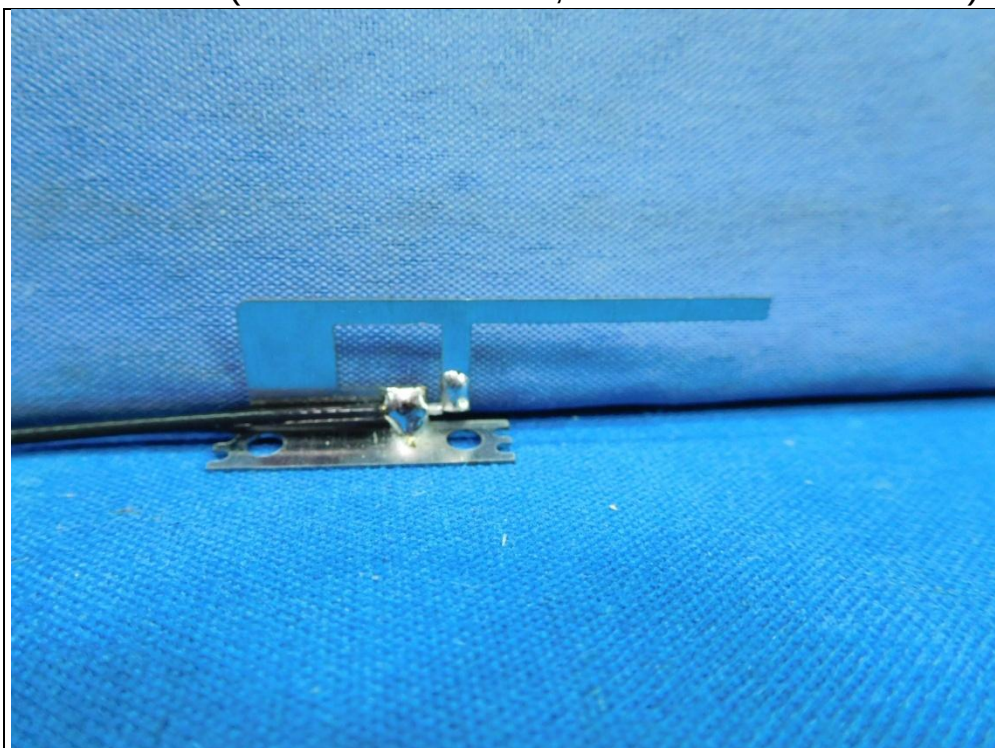
Antenna 24 (Brand: LYNWAVE ; Model: ALA120-052024)
