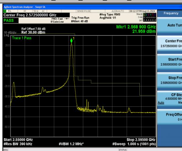
Band7 20MHz 16QAM 21350 1RB#99
