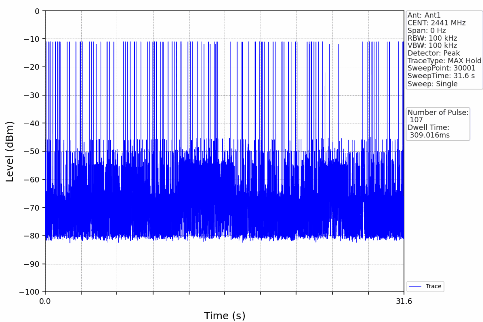
GFSK_DH5_HOPP_Ant1_NTNV
