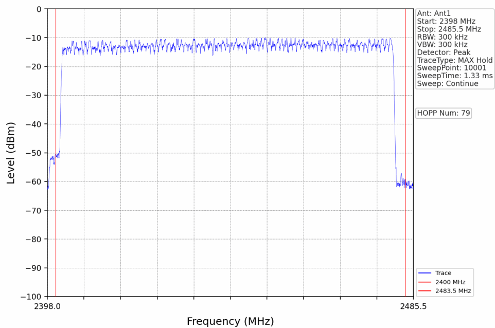
\pi/4 -DQPSK_2DH5_HOPP_Ant1_NTNV
