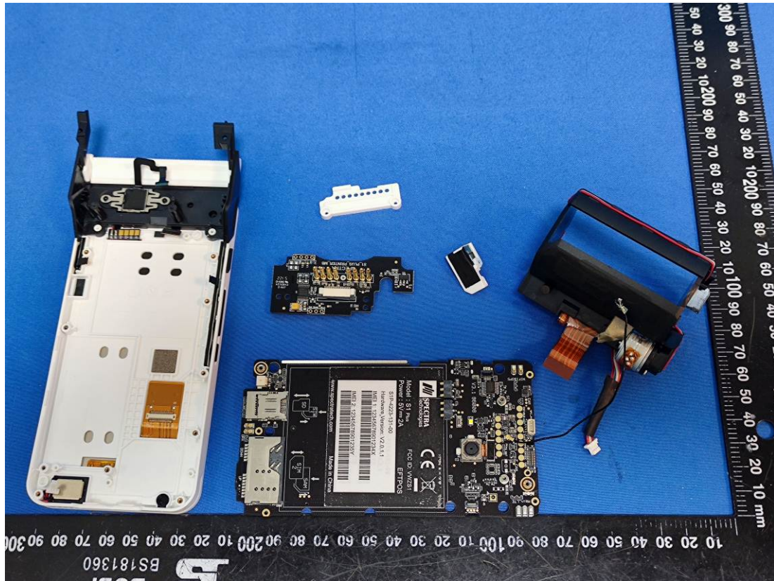
NFC Antenna-1
