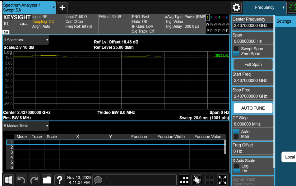
NTNV-11G-Ant1-2437
