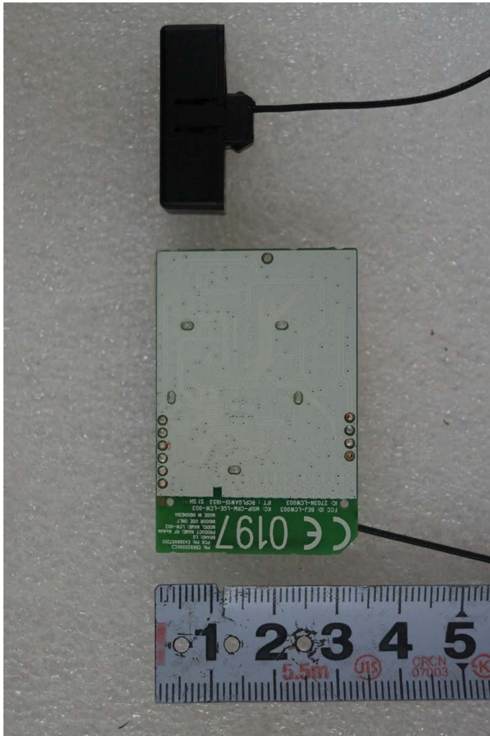
<Wi-Fi module Section -2>
