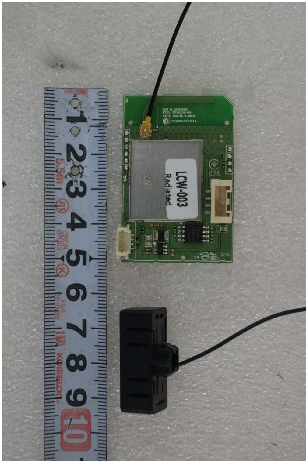
<Wi-Fi module Section -1>
