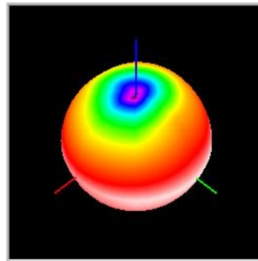
GSM900 -TIS
