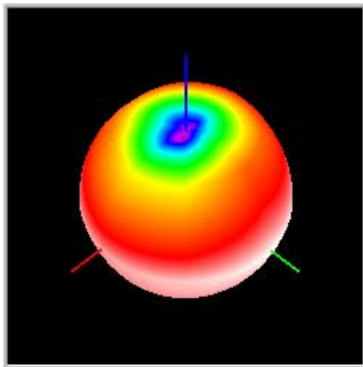
GSM900 -TRP
