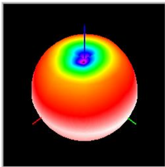
GSM850 -TRP
