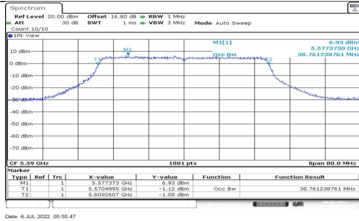
11AX40SISO_Ant1_5590
