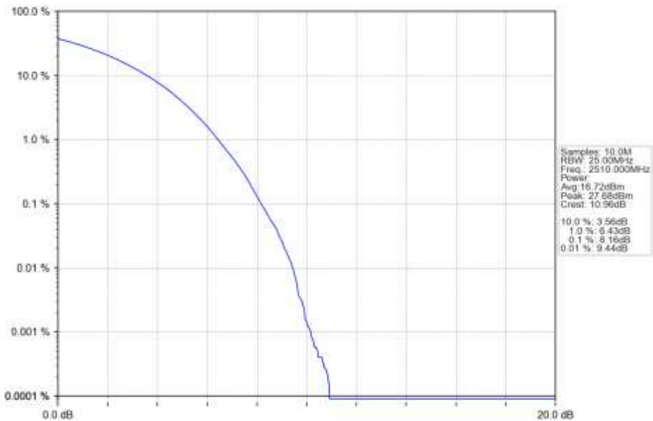
n7_15kHz_SISO_NTNV_20MHz_CP-OFDM_256_QAM_2510MHz_Outer_Full_Ant1
