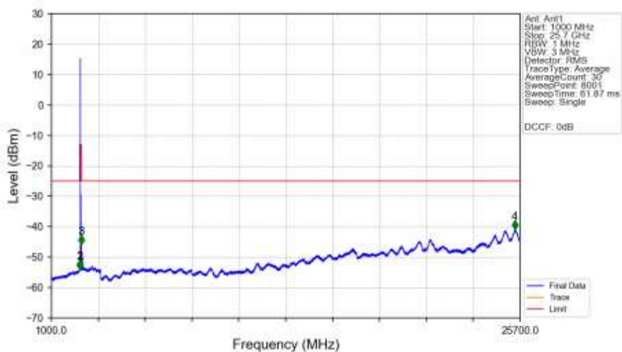
n7_15kHz_SISO_NTNV_20MHz_DFT-s-OFDM_QPSK_2535MHz_Edge_1RB_Left_Ant1
