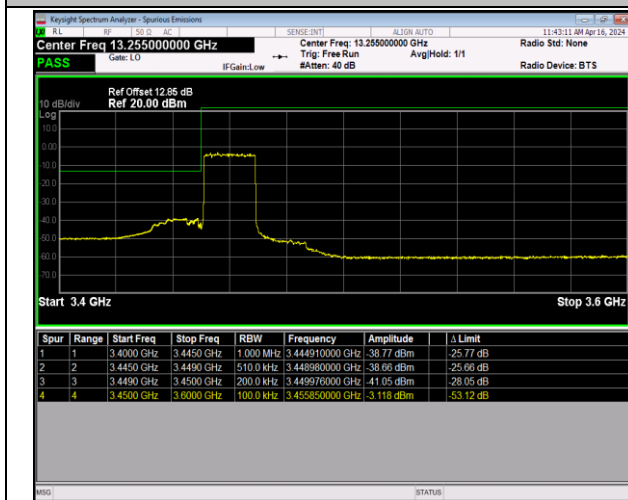
Band42_20MHz_QPSK_42190_100RB#0
