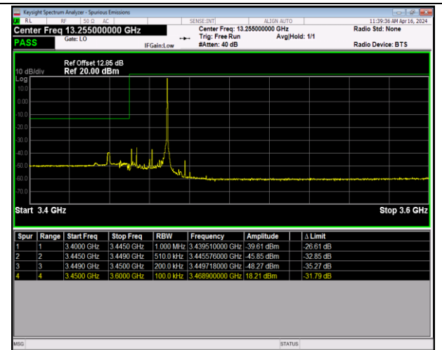
Band42_20MHz_QPSK_42190_1RB#99
