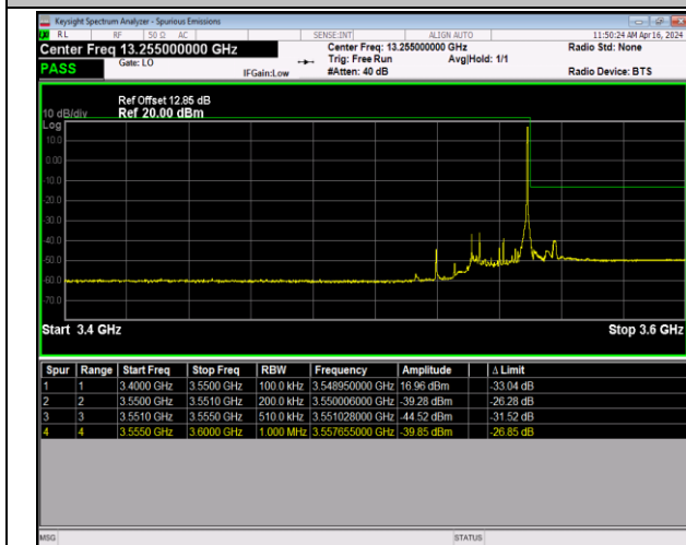
Band42_20MHz_QPSK_42990_1RB#99
