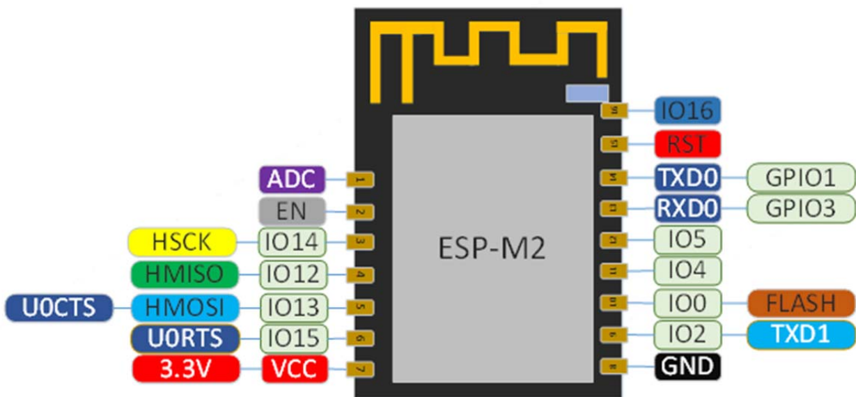
图 2.2 ESP-M2 Definition for Pins
