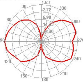
2400.000MHz E1
