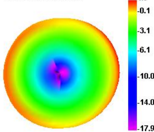
2450.000MHz
