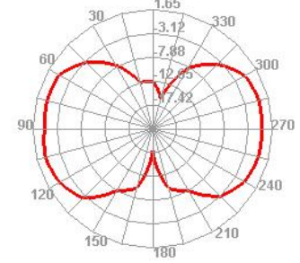
2500.000MHz E2
