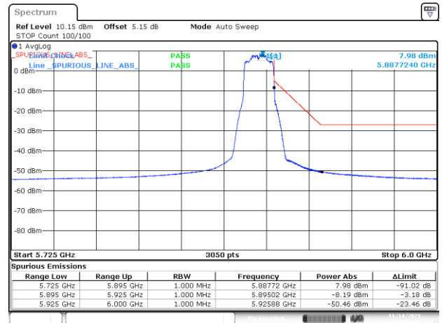
BE-NR-HIGH, MIMO-A, 802.11ax20-MCS0, Ch177
