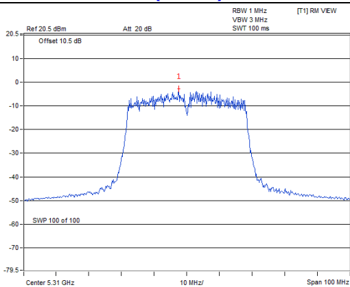
802.11ac (40MHz)_Chain 0 / CH62
