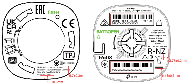
尺寸图
