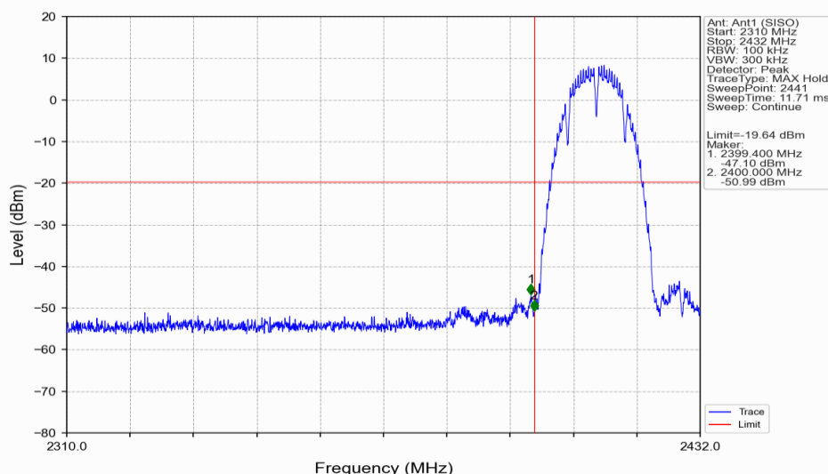
802.11b_LCH_2412MHz_Ant1 (SISO)_NTNV
