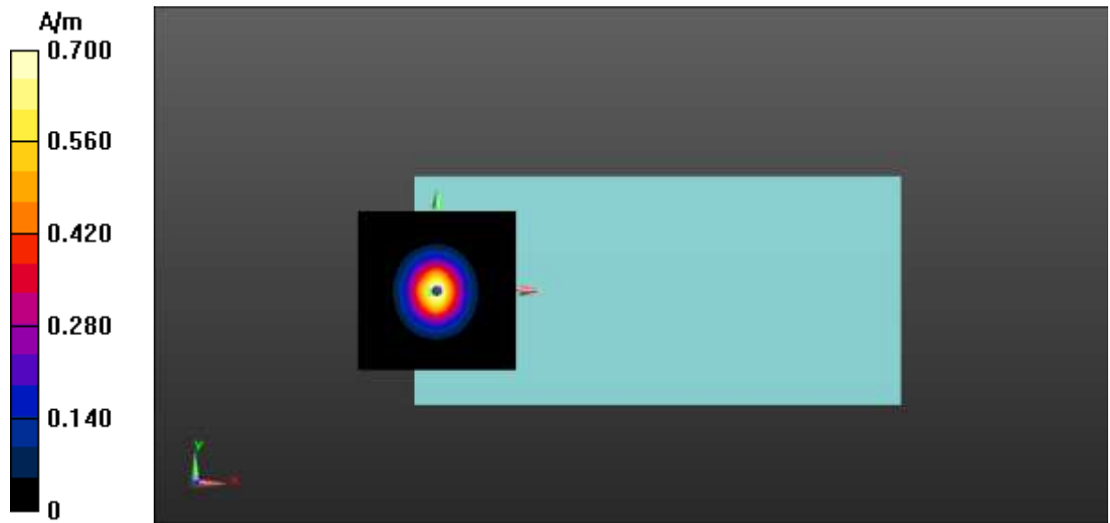
Fig A.9 T-Coil WCDMA B5
