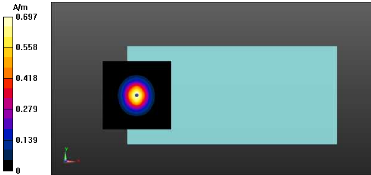
Fig A.5 T-Coil WCDMA B2
