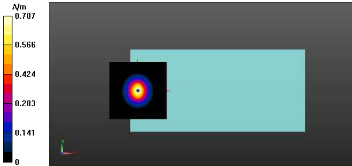
Fig A.7 T-Coil WCDMA B4
