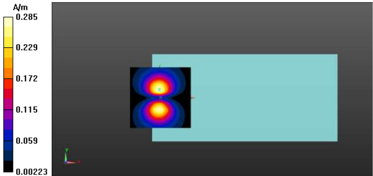
Fig A.10 T-Coil WCDMA B5
