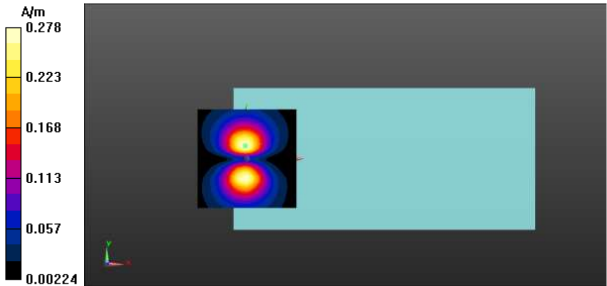
Fig A.8 T-Coil WCDMA B4
