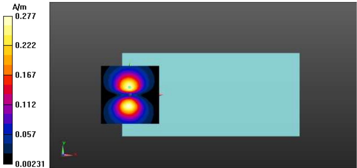
Fig A.6 T-Coil WCDMA B2
