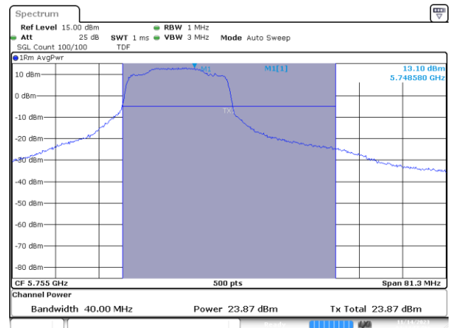
MIMO B-802.11ax/be40-CH151-5755MHz-MCS0 20m
