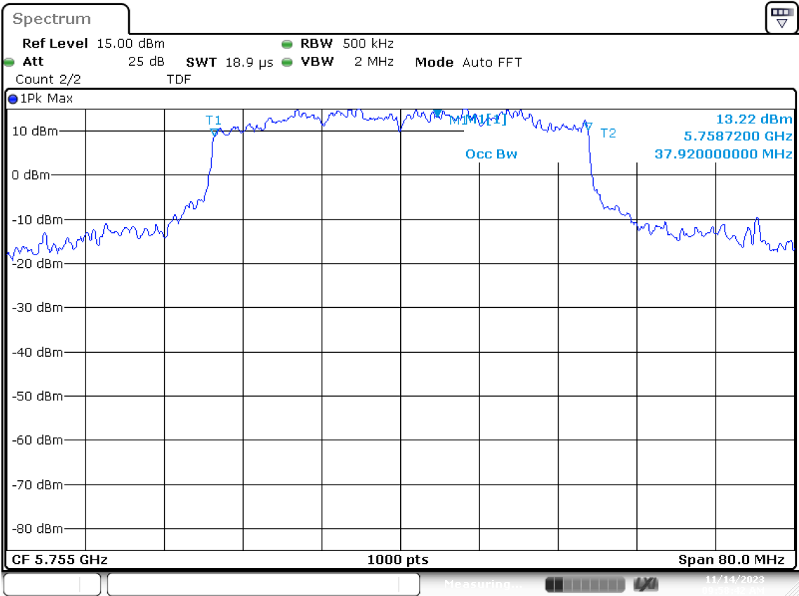
SISO B-802.11ax/be40-CH151-5755MHz-MCS0
