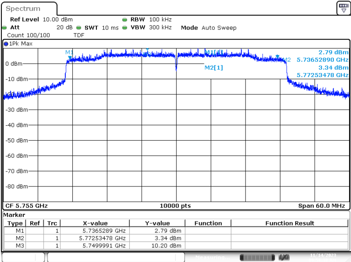
SISO B-802.11ax/be40-CH151-5755MHz-MCS0
