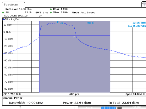
MIMO A-802.11ax/be40-CH151-5755MHz-MCS0 20m
