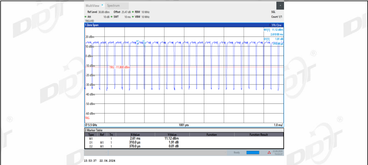
11BE20MIMO_Ant2_5500
