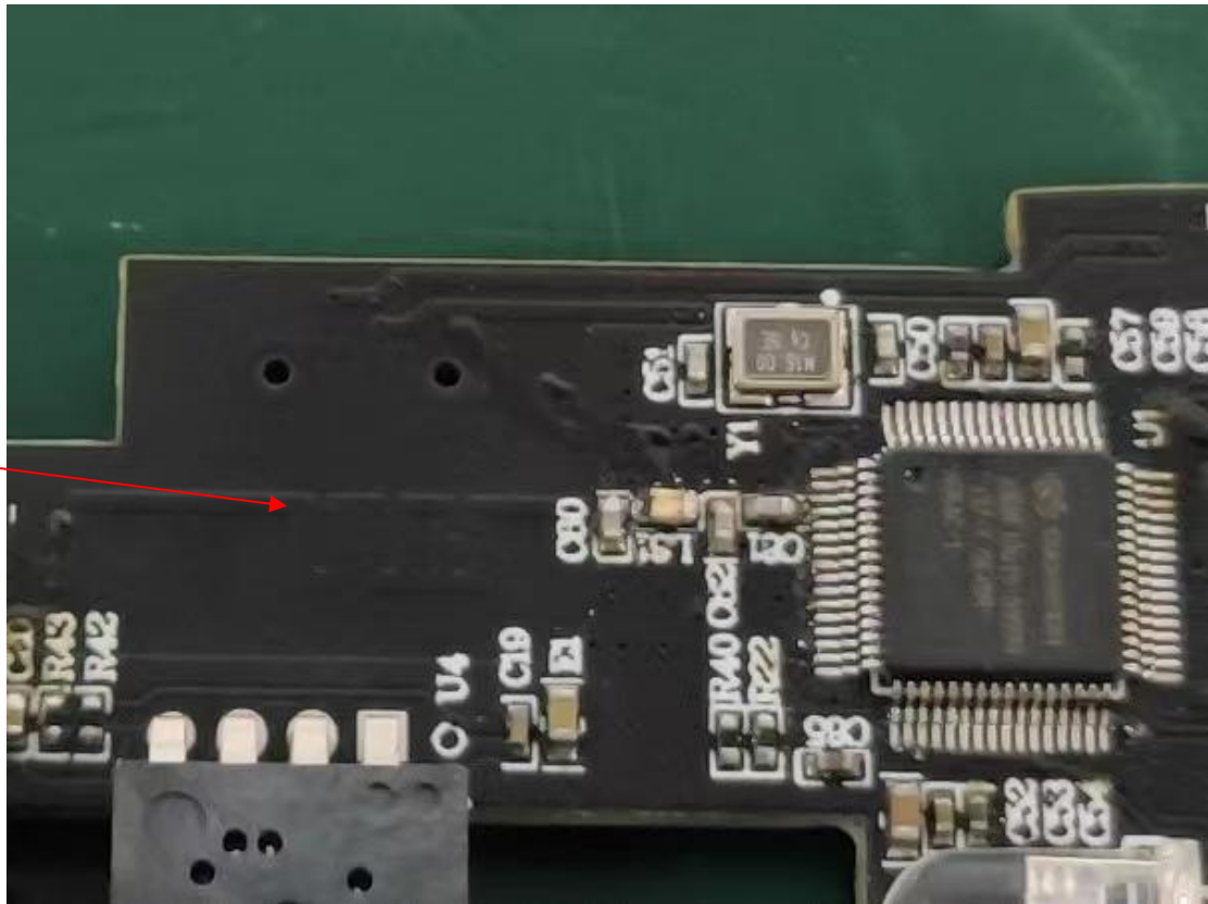
Internal photos M/N: Serafim M1 Pro
