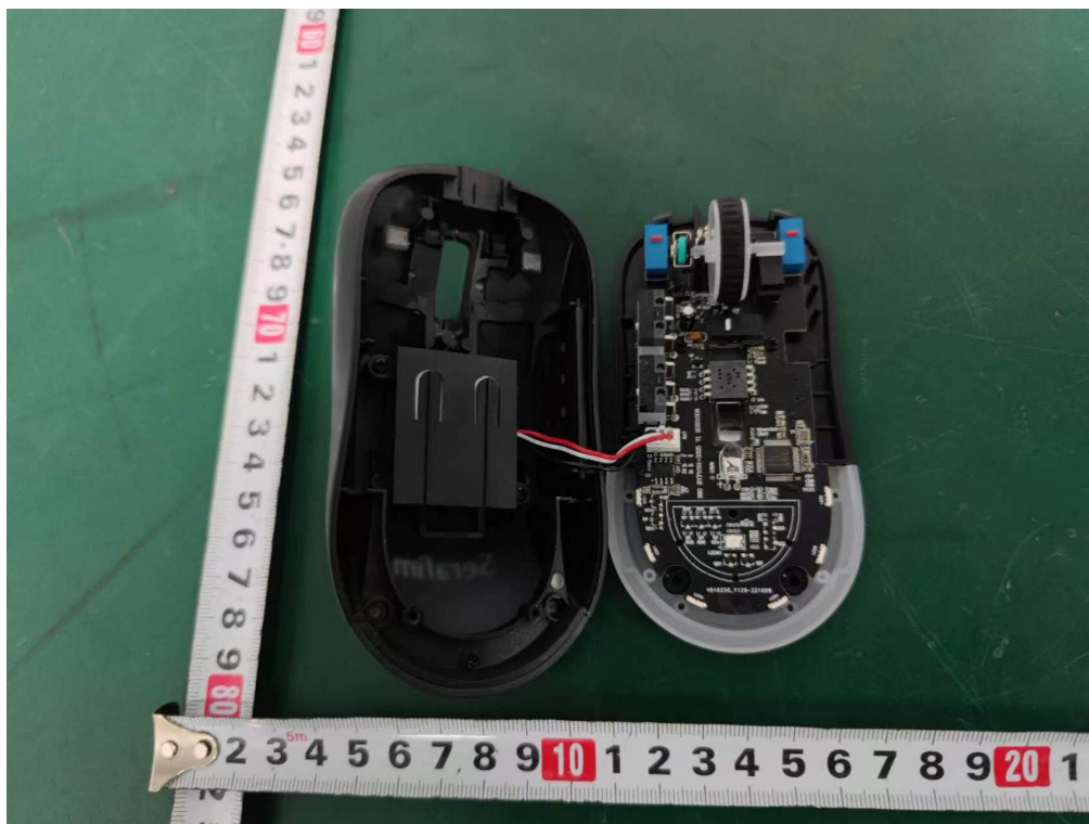
Internal photos M/N: Serafim M1 Pro
