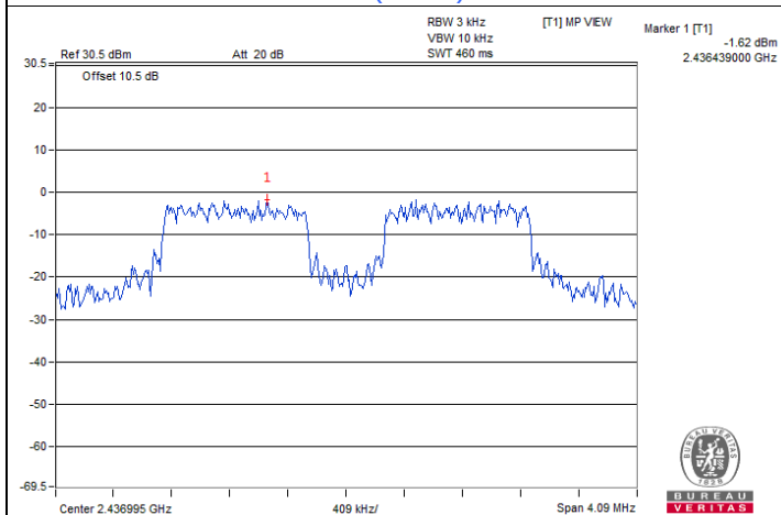
20 MHz Preamble 802.11ax (RU26) : CH 6
