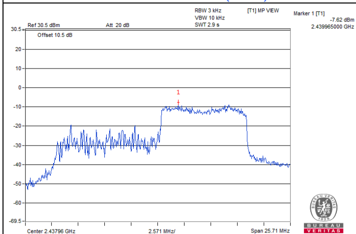
20 MHz Preamble 802.11ax (RU106) : CH 6
