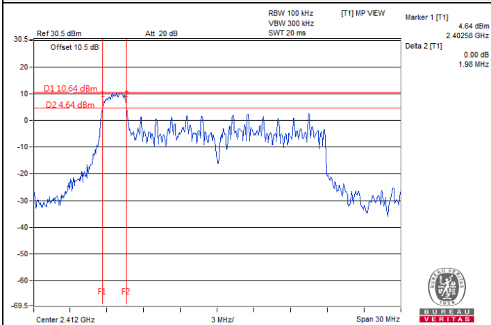
20 MHz Preamble 802.11ax (RU26) : CH 1
