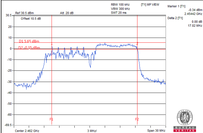
20 MHz Preamble 802.11ax (RU106) : CH 11
