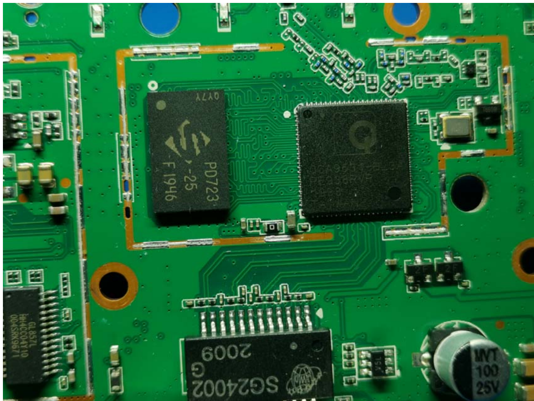
GL-X750V2
