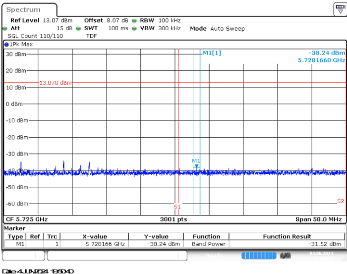
BE-NR-HIGH, SISO-A, 802.11ax/be160-MCSO, Ch114
