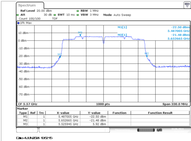
SISO A-802.11ac-160MHz-114-5570-VHT0 -26dB
