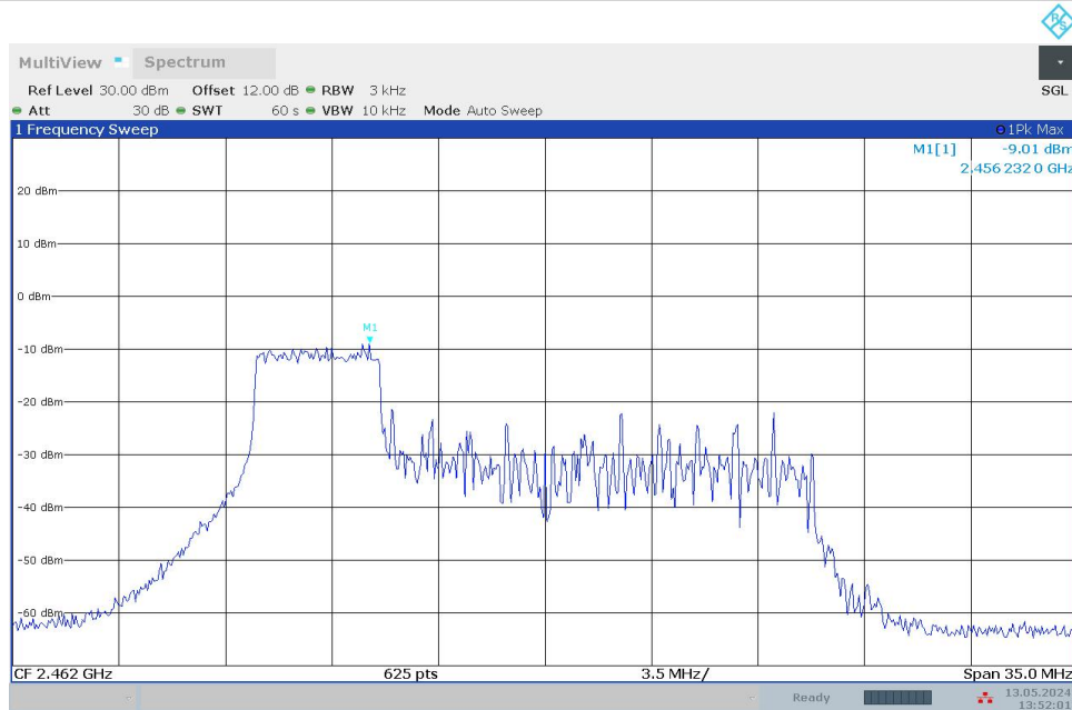
11BE20MIMO_Ant1_2462_52Tone_RU40
