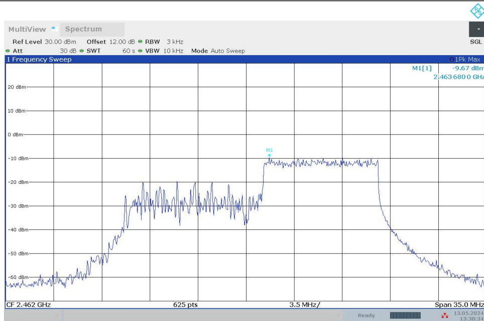
11BE20MIMO_Ant1_2462_26Tone_RU0
