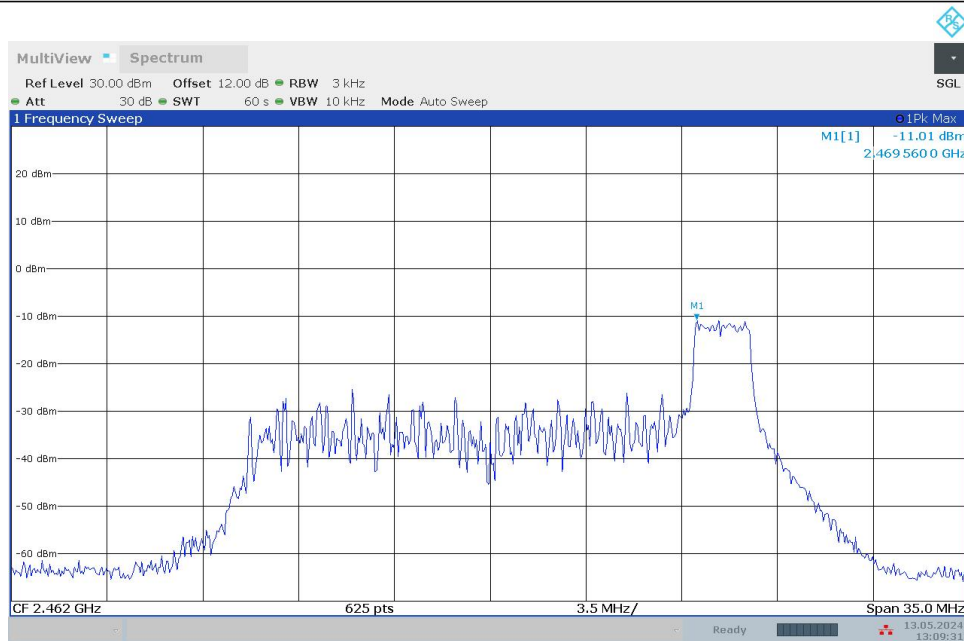
11BE20MIMO_Ant0_2462_52Tone_RU37
