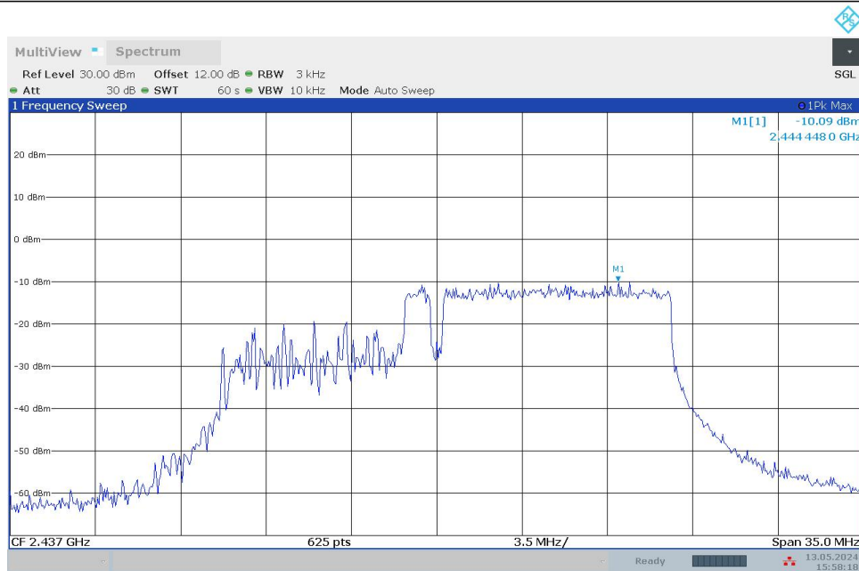
11BE20MIMO_Ant1_2437_52+26_OFDMA_1
