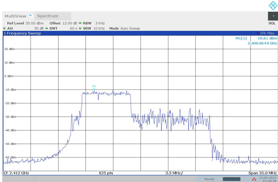
11BE20MIMO_Ant0_2412_52+26_OFDMA_3
