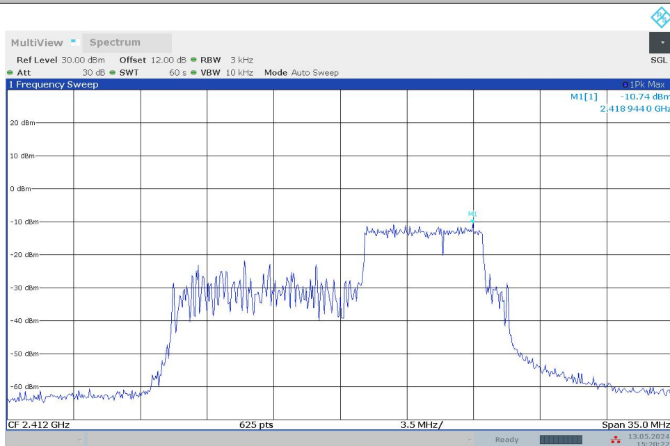
11BE20MIMO_Ant1_2412_52+26_OFDMA_3
