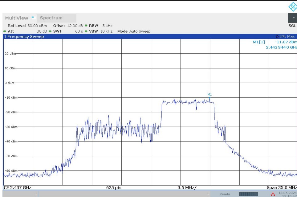
11BE20MIMO_Ant1_2437_106+26_OFDMA_1
