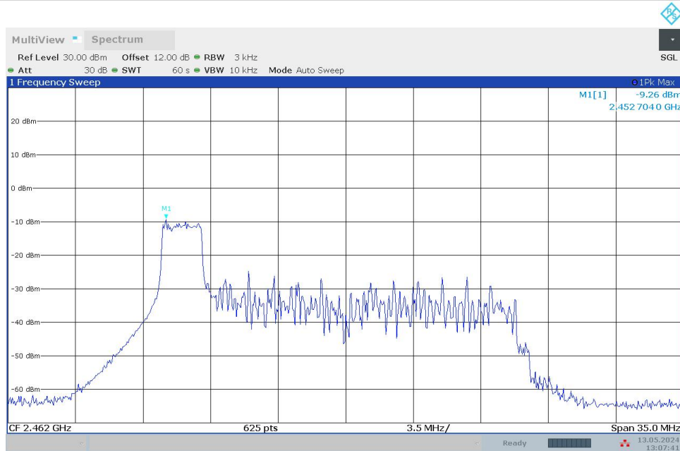
11BE20MIMO_Ant0_2462_26Tone_RU8
