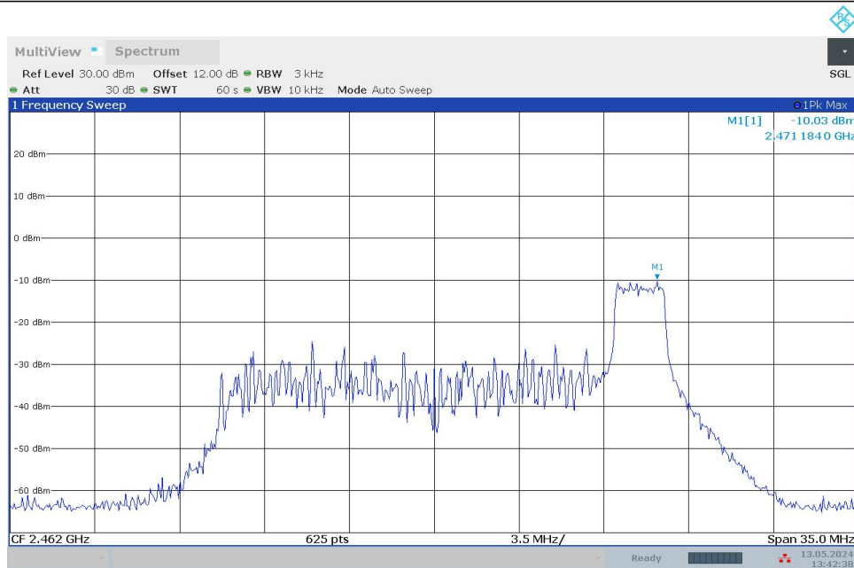
11BE20MIMO_Ant1_2462_52Tone_RU37
