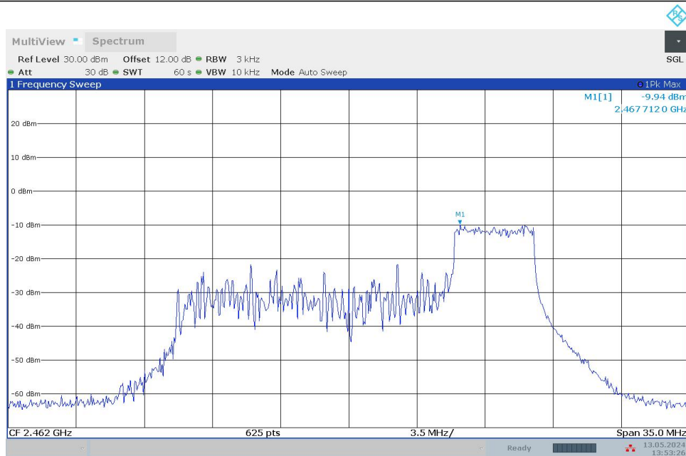
11BE20MIMO_Ant1_2462_106Tone_RU53
