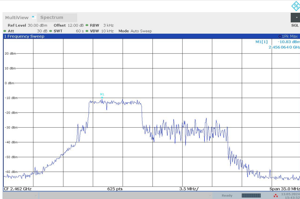
11BE20MIMO_Ant0_2462_52+26_OFDMA_3
