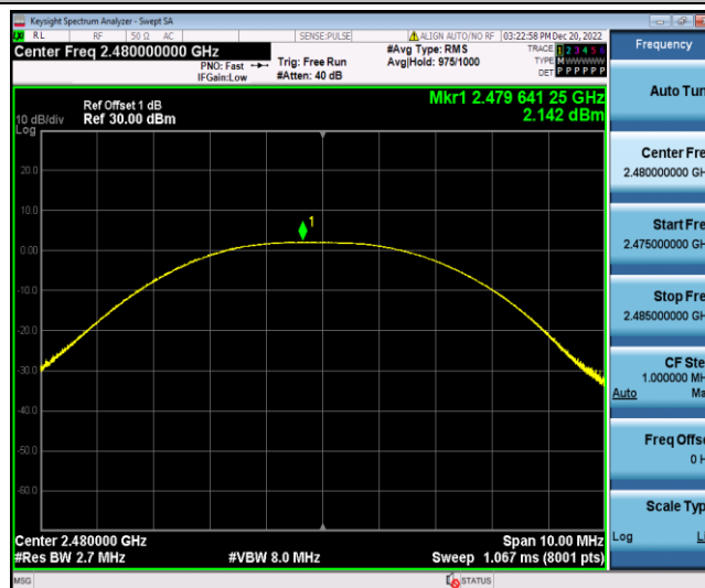
BLE_2Mbps_Ant1_2480
