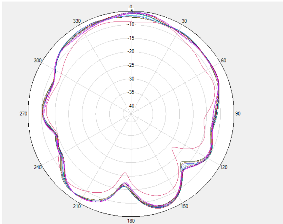
2.4G WIFI&BT Phi=0deg
