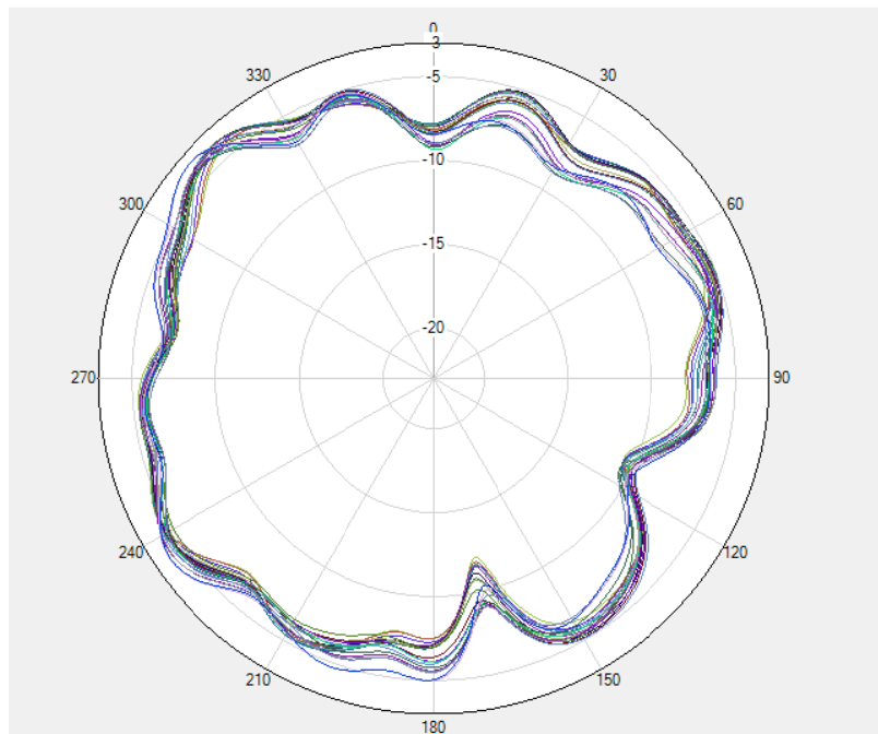
GPS Phi=90deg
