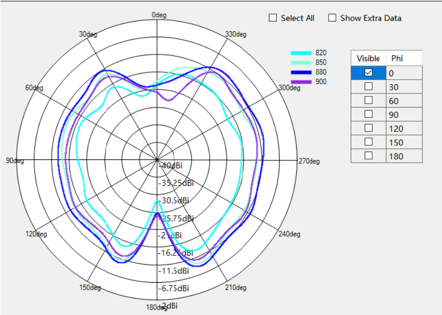
GSM850/WCDMA B5/LTE B5/B20 \Phi=0^\circ
