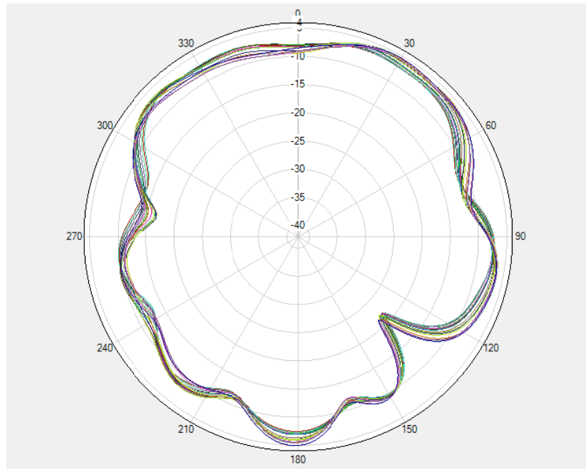
GPS Phi=0deg
