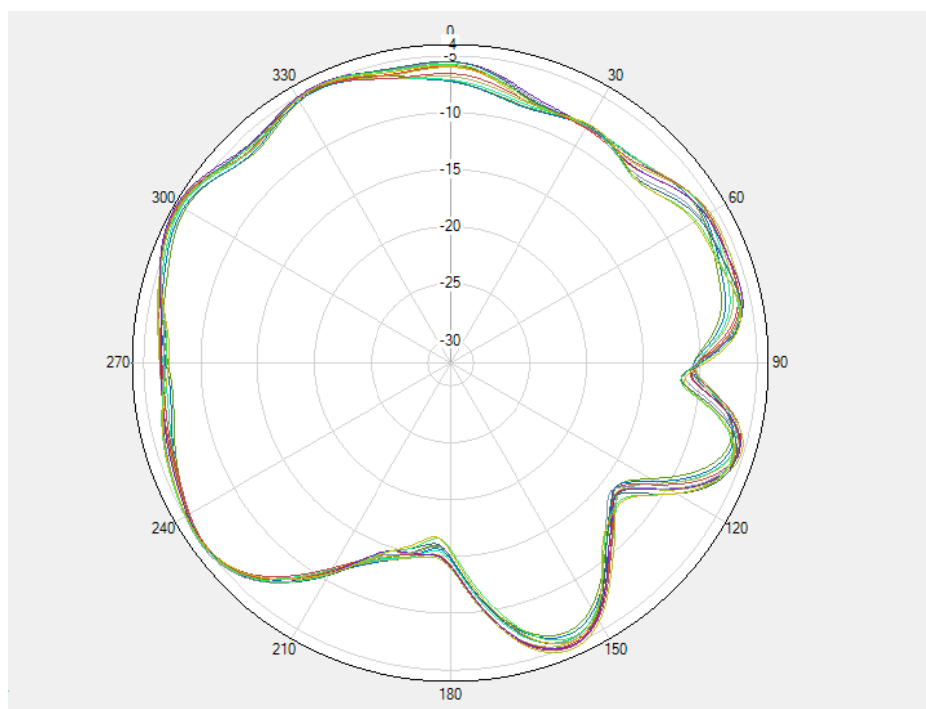
2.4G WIFI&BT Phi=90deg
