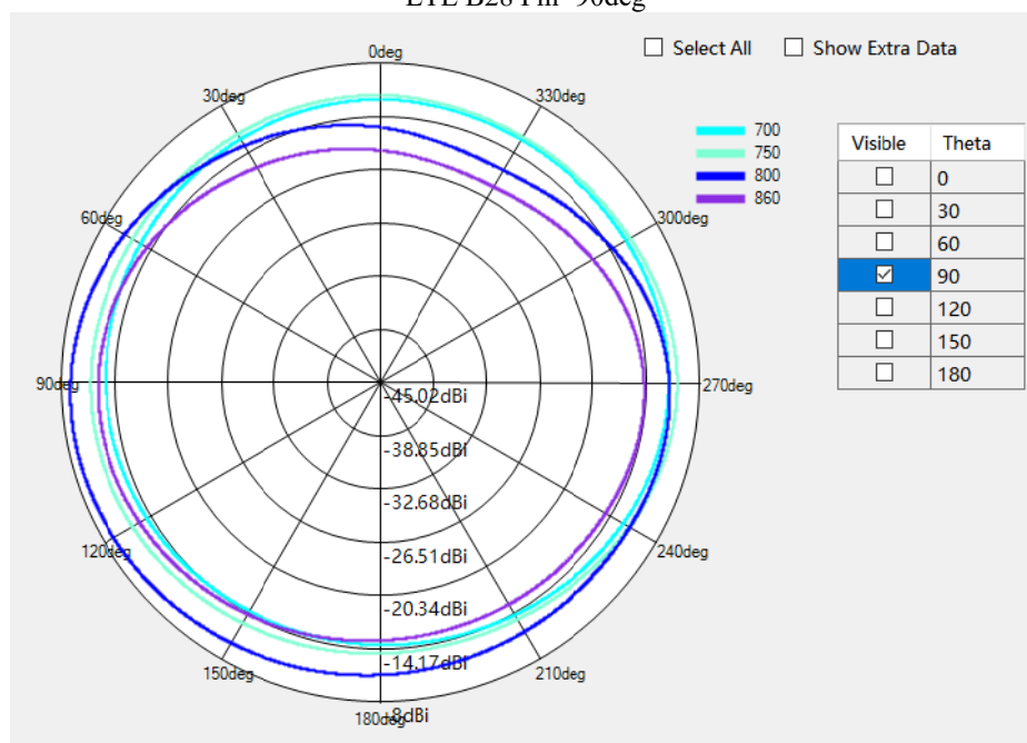
LTE B28 Theta=90deg
