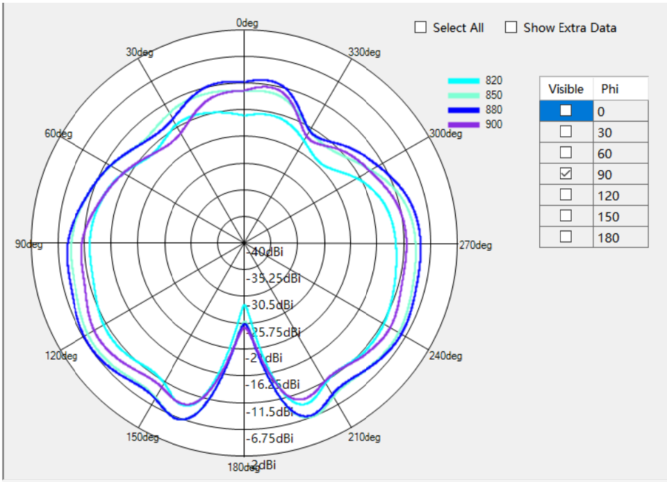
GSM850/WCDMA B5/LTE B5/B20 \Phi=90^\circ
