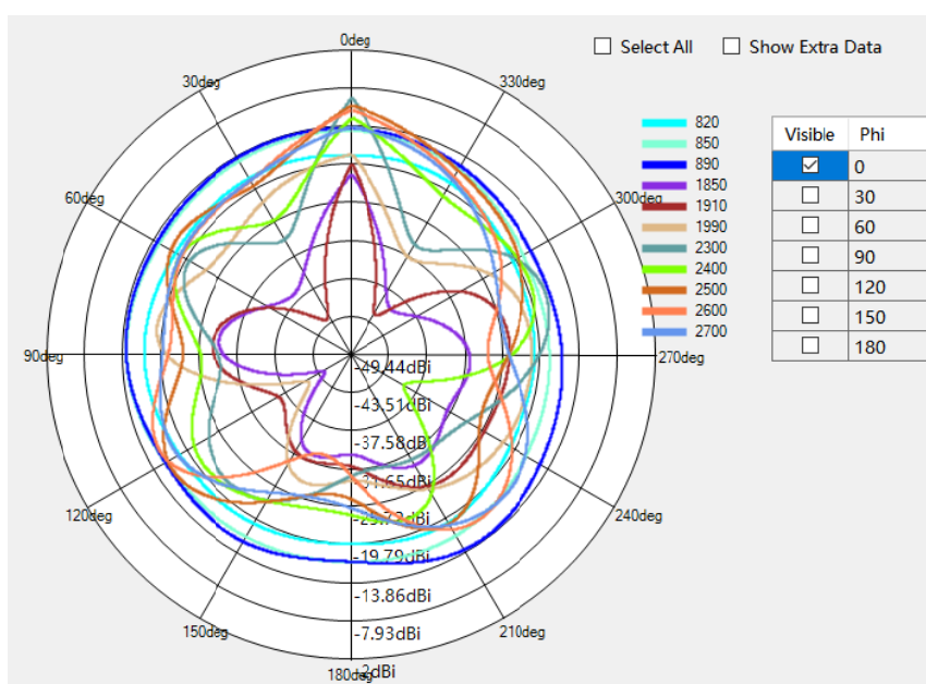
GSM850/PCS / WCDMA B1/B2/B5 / LTE B1/B2/B5/B7/B38/B41 Phi=0deg
