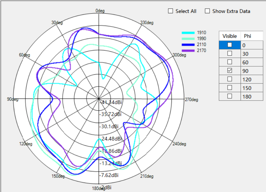
LTE B1Phi=90deg
