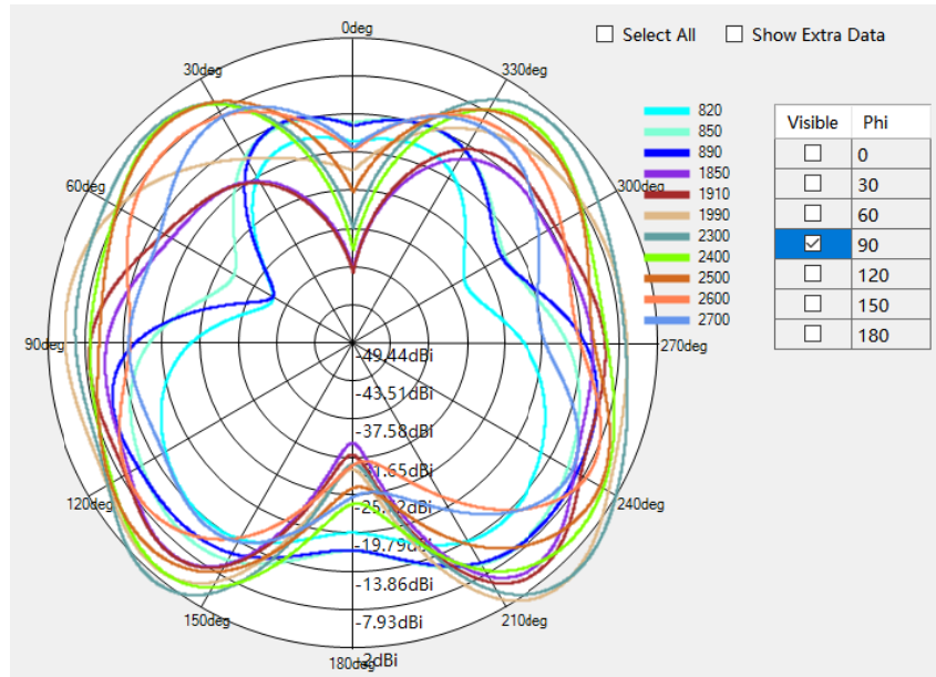
GSM850/PCS / WCDMA B1/B2/B5 / LTE B1/B2/B5/B7/B38/B41 Phi=90deg
