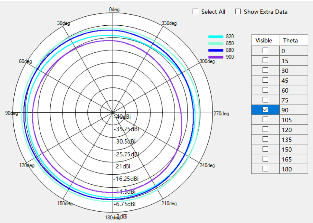
GSM850/WCDMA B5/LTE B5/B20 Theta=90deg
