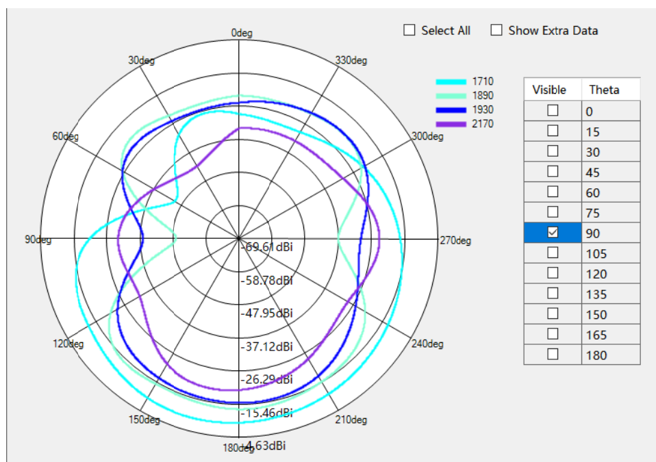
DCS1800/PCS1900/WCDMA B1/B2/B4/LTE B1/2/3/4 Theta=90deg
