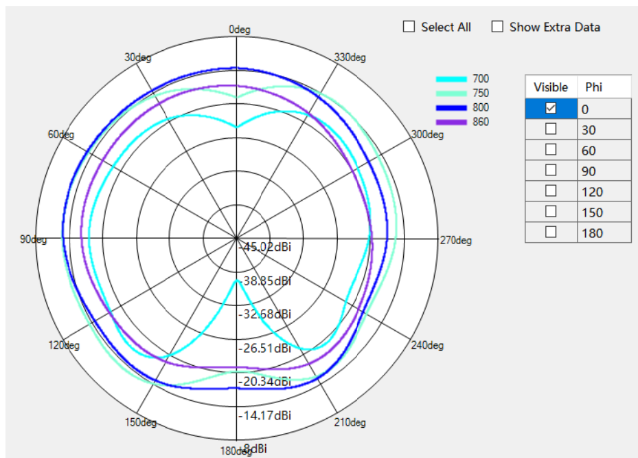
LTE B28 Phi=0deg
