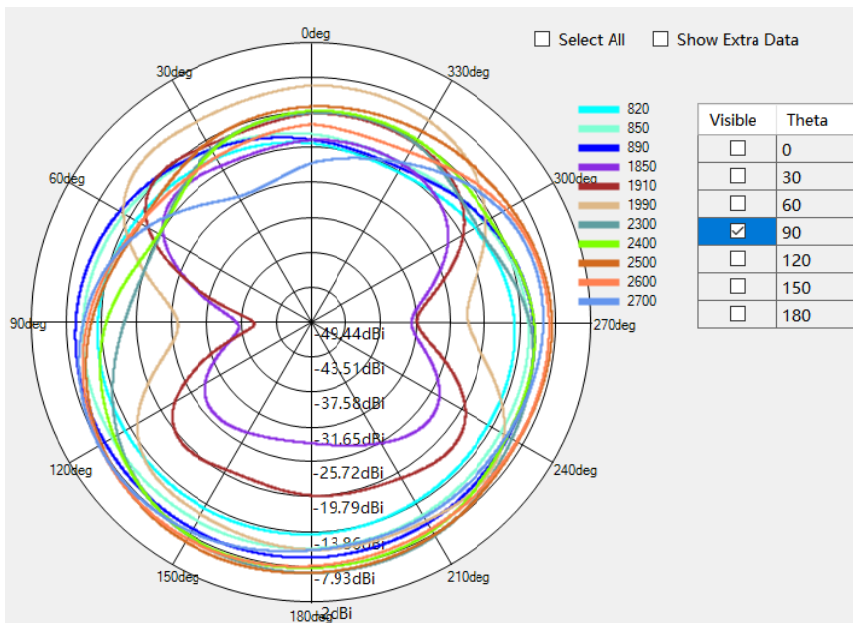
GSM850/PCS / WCDMA B1/B2/B5 / LTE B1/B2/B5/B7/B38/B41 Theta=90deg
