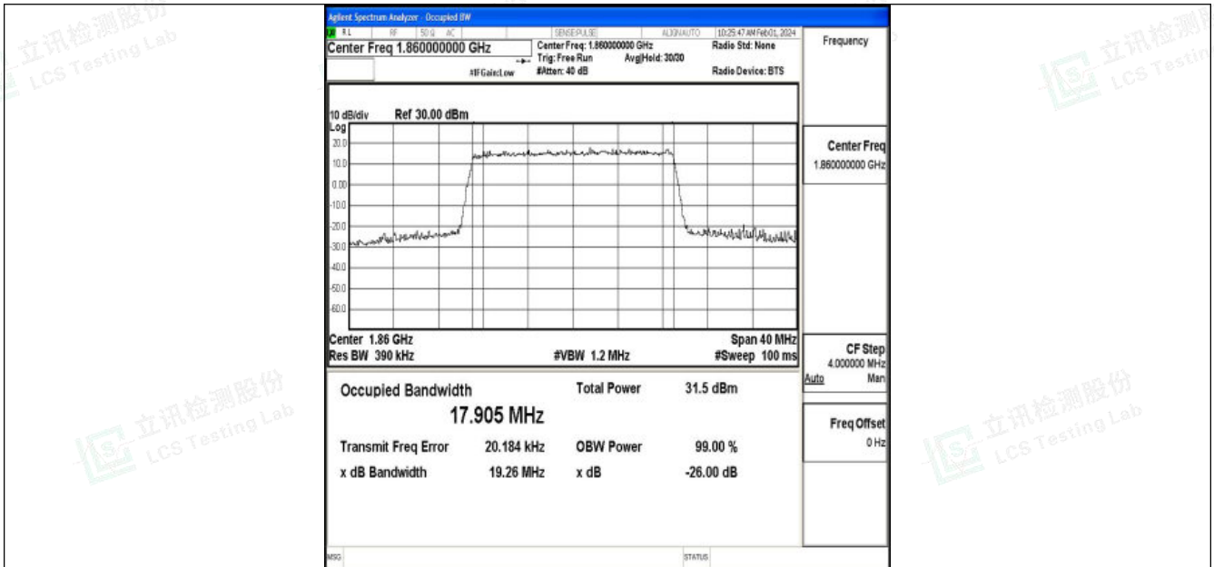
Band2-20MHz-QPSK-18700-100RB#0-PASS
