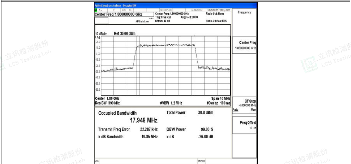
Band2-20MHz-16QAM-18700-100RB#0-PASS
