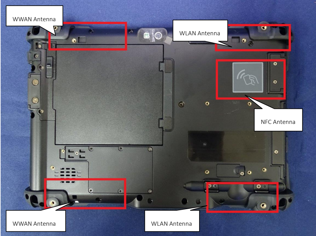
(71) EUT Photo
