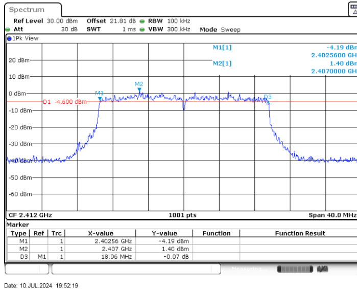
11BE20MIMO_Ant2_2412
