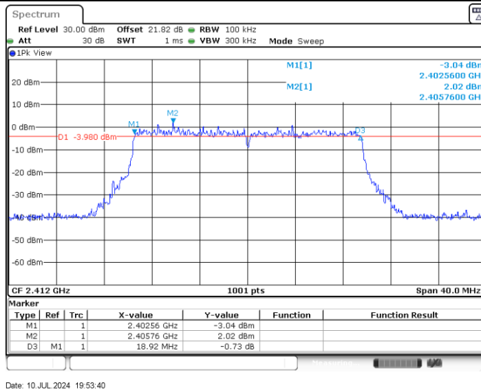
11BE20MIMO_Ant2_2412
