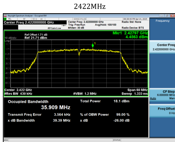
802.11n(HT40)_ANT2
