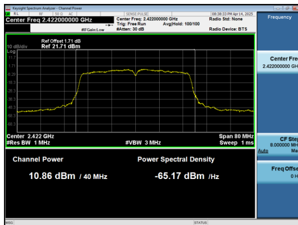
802.11n(HT40)_ANT2_MIMO
