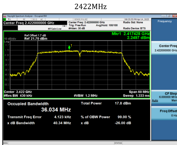
802.11n(HT40)_ANT1
