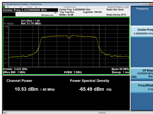
802.11n(HT40)_ANT1_MIMO
