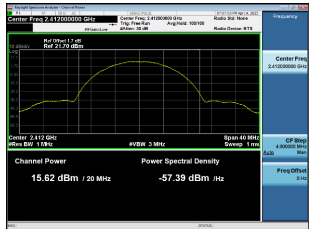
802.11b_ANT 2
