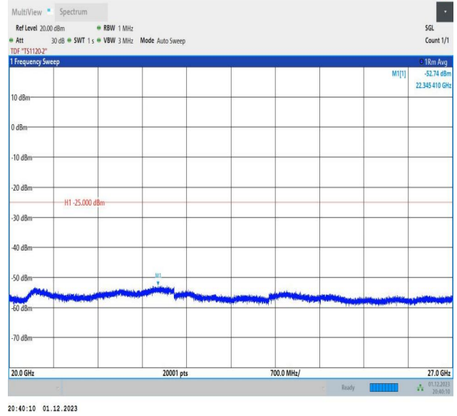
7-7-20MHz-20MHz-QPSK-QPSK-20850-21048-100RB#0-100 RB#0-20000~27000MHz-PASS
